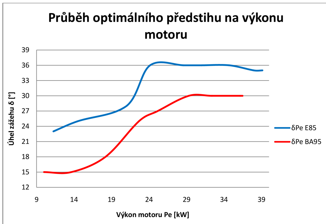
Graf. 2 Průběh optimálního předstihu v závislosti na výkonu motoru pro paliva BA95 a E85
