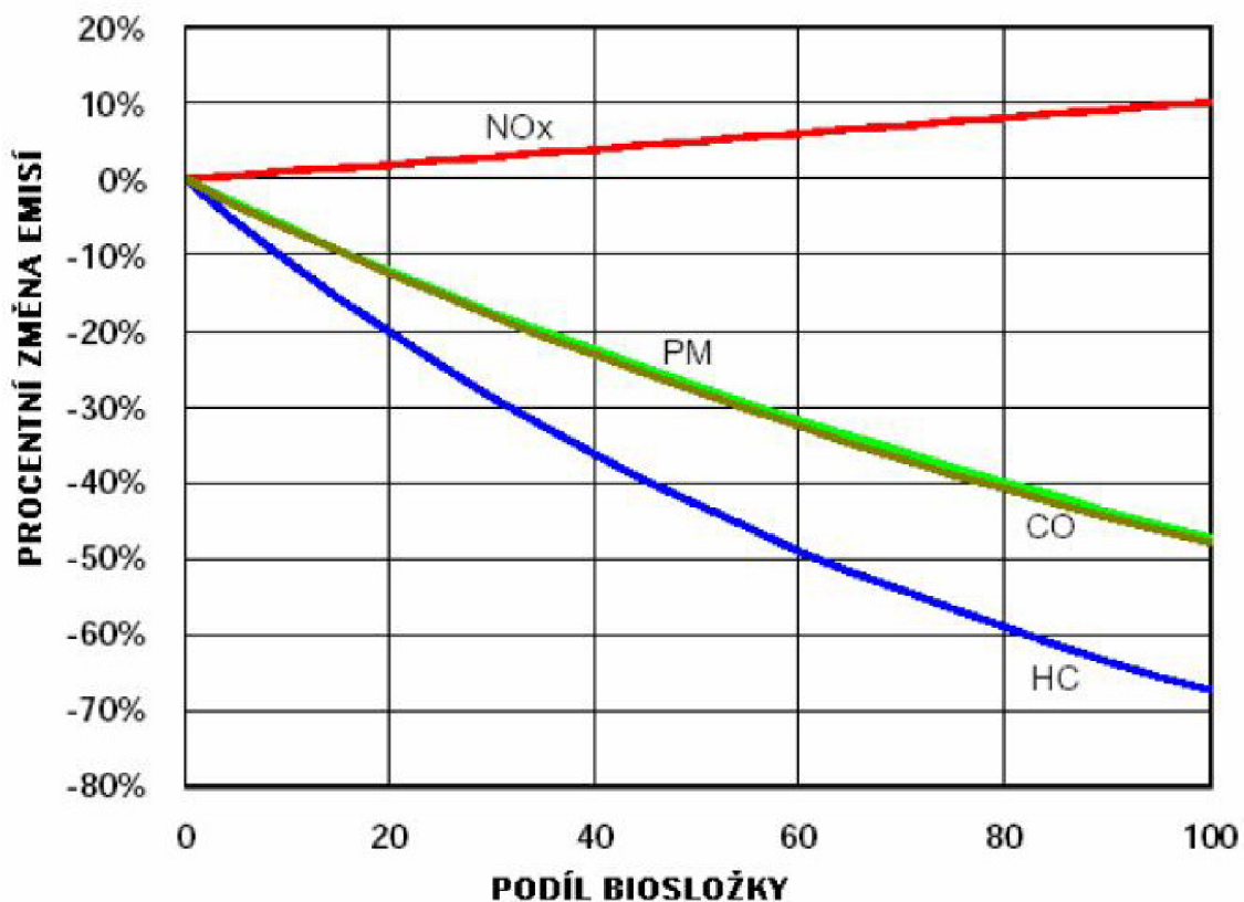
Obr. 10 Změna limitních prvků výfukových plynů po přidání biosložek do fosilních paliv [16]
