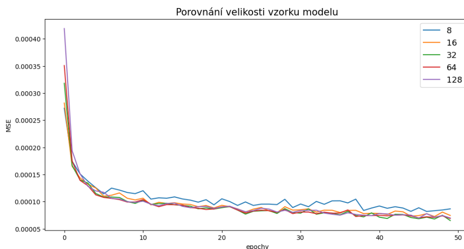
Obrázek 3.24: Porovnání chyby modelů v závislosti na velikosti vzorku
