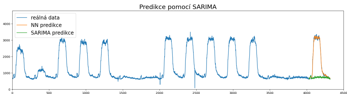
Obrázek 5.7: Predikce datasetu s1 pomocí SARIMA algoritmu
