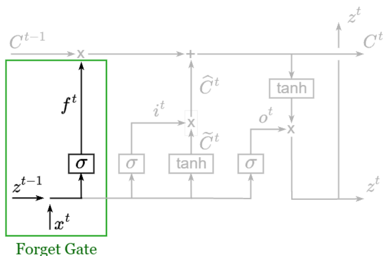
Obrázek 2.8: Forget Gate
