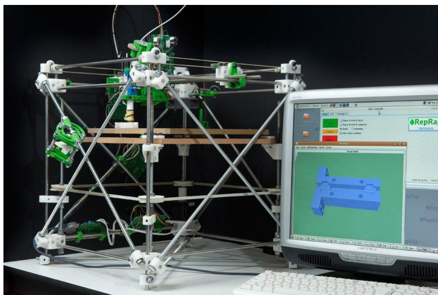
Obr. 2-7 Tiskárna Darwin. [17]
