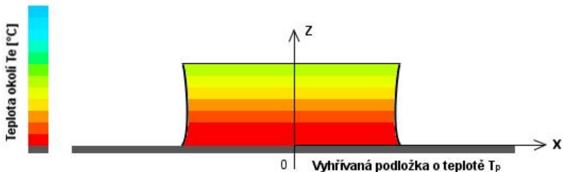
Obr. 2-23 Deformace spodních vrstev.
