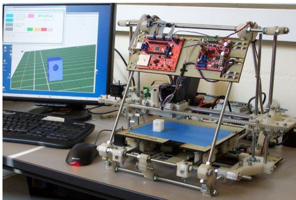
Obr. 2-8 Tiskárna Mendel. [18]
