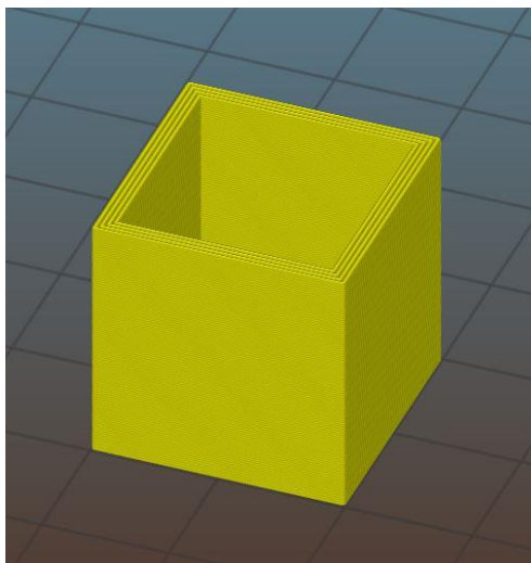
Obr. 5-6 Díl pro testování deformace spodních vrstev
