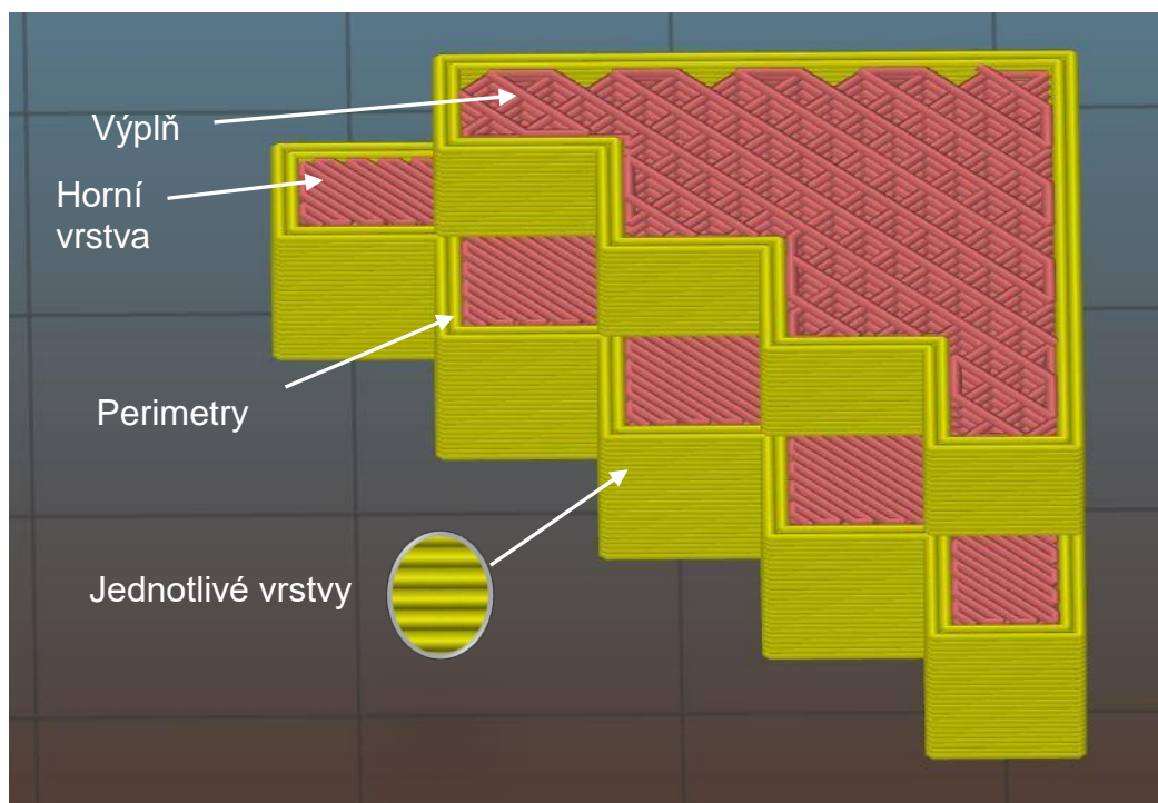
Obr. 2-10 Stavební prvky.
