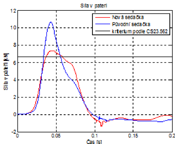
Obrázek 17: Porovnání sil působících do páteře pro původní a nově navrženou sedačku letounu TL-Stream [24]
