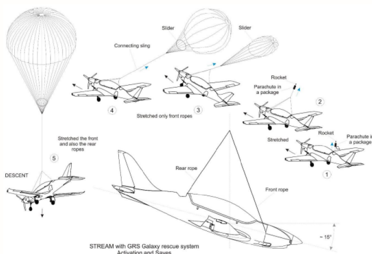
Obrázek 16: Schéma padákového systému TL-Ultralight [22]
