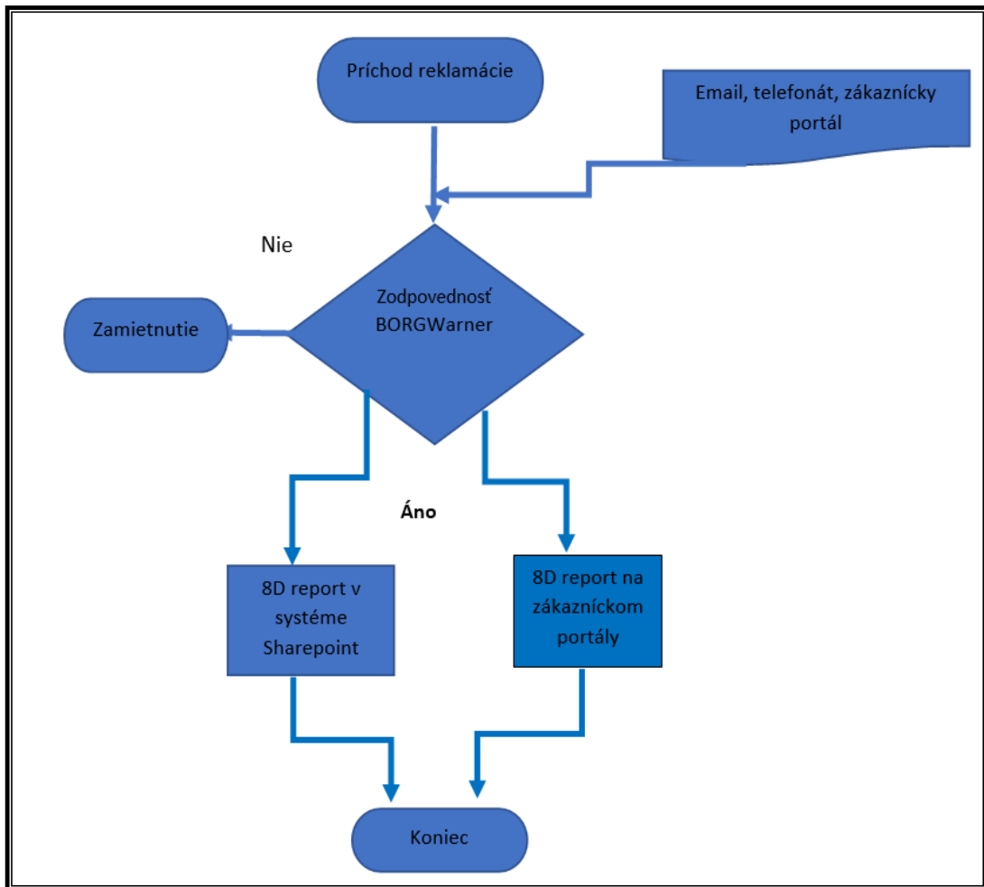
Obr. 3.8 Vývojový diagram
