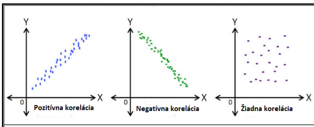
Obr. 2.6 Druhy korelácie
