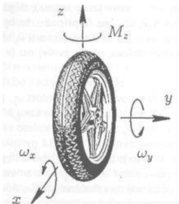
Obr. č. 4.1 – Vznik gyroskopického momentu [16]
