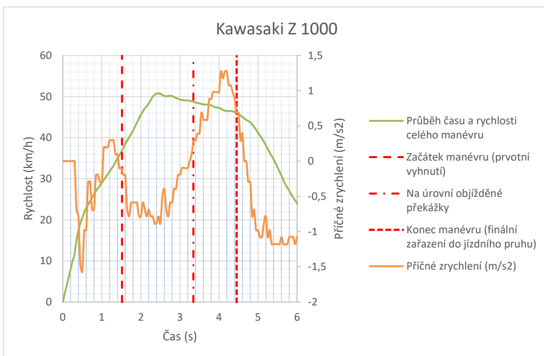
Graf č. B.10 – Průběh času a rychlosti při průjezdu slalomem Kawasaki Z 1000
