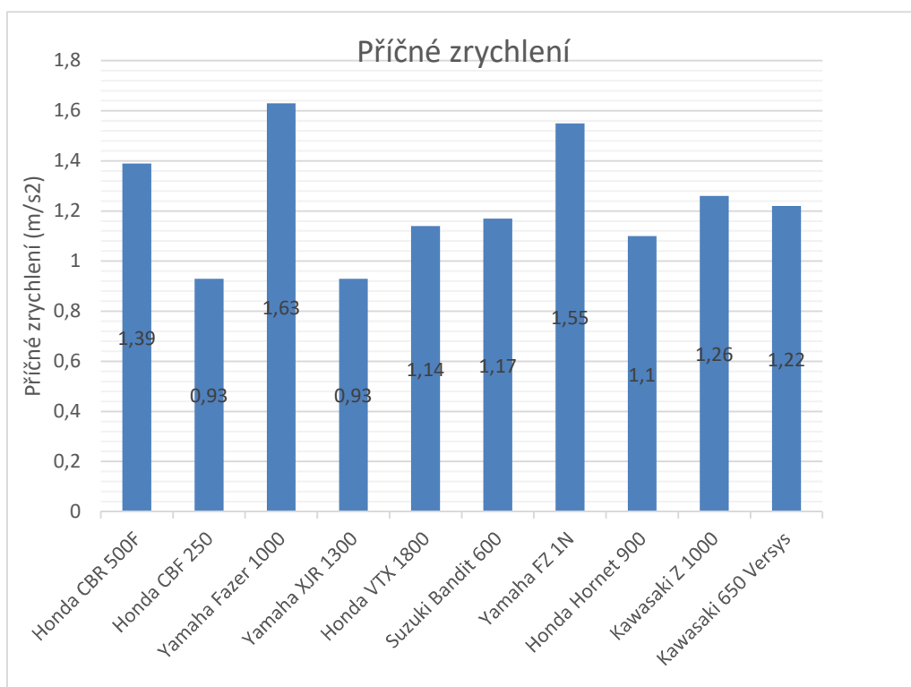
Graf. č. 8.2 – Hodnoty příčného zrychlení pro daný motocykl vypočítané vyjádřením ze vorce (8.2)
