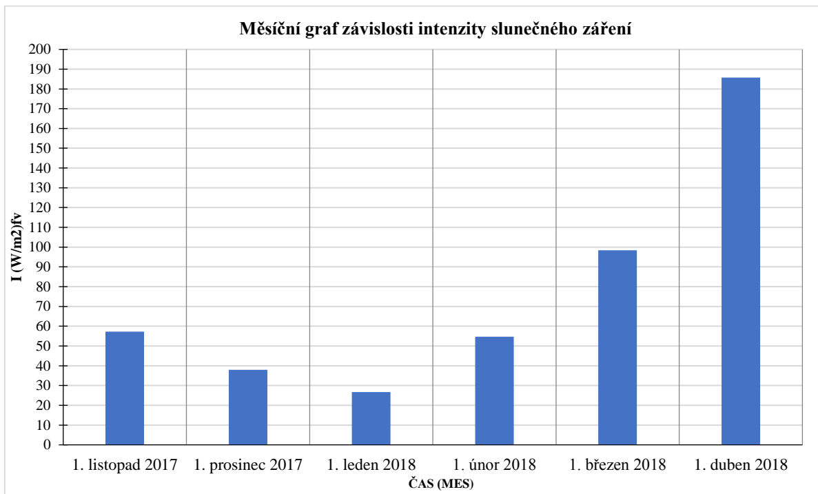
Obr. 5.10 Měsíční graf závislosti intenzity slunečního záření
