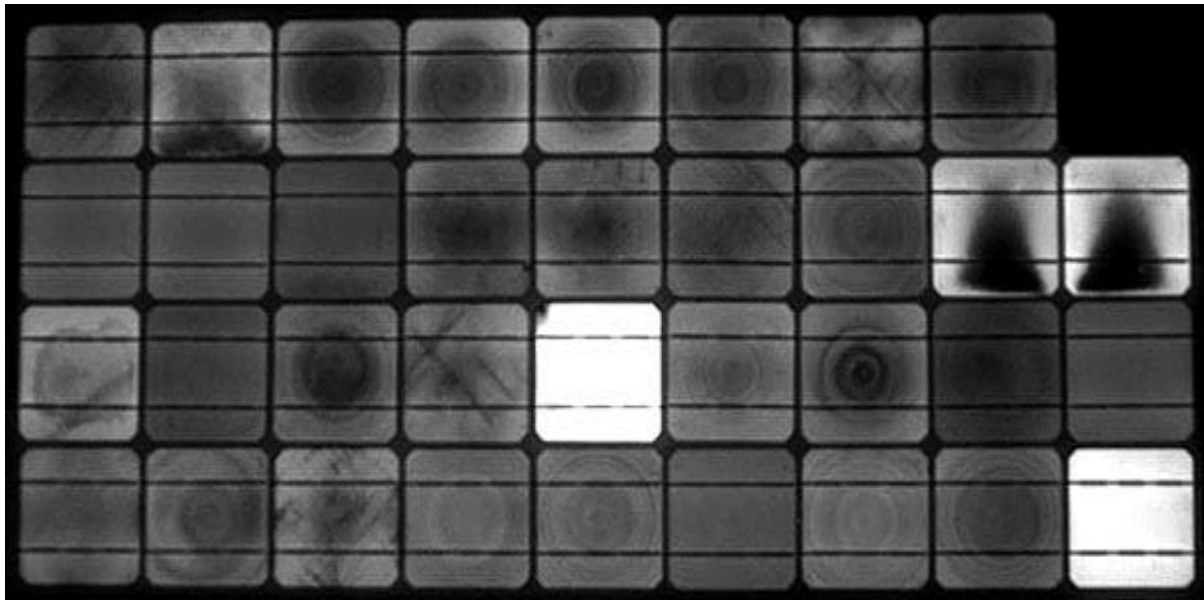
Obr. 4.10 Panel s vadnými fotočlánky [14]
