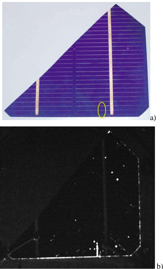
Obr. 4.9 a,b Mechanické poškození fotočlánků a) Zřetelní obraz b) Fotoluminiscenční obraz [14]
