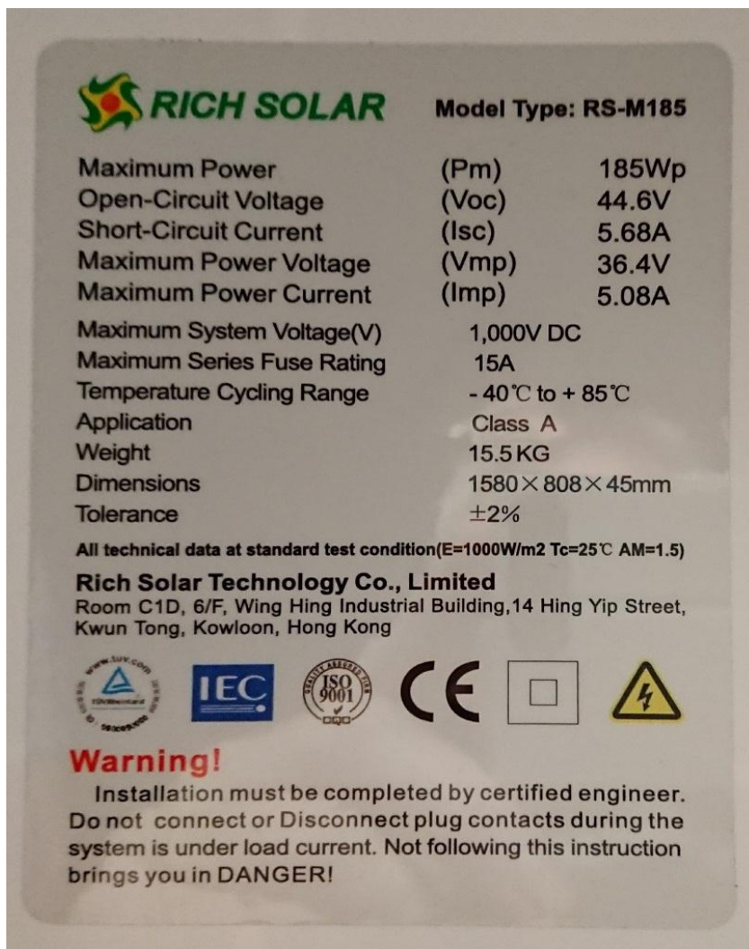
Obr. 5.13 Štítek panelu
