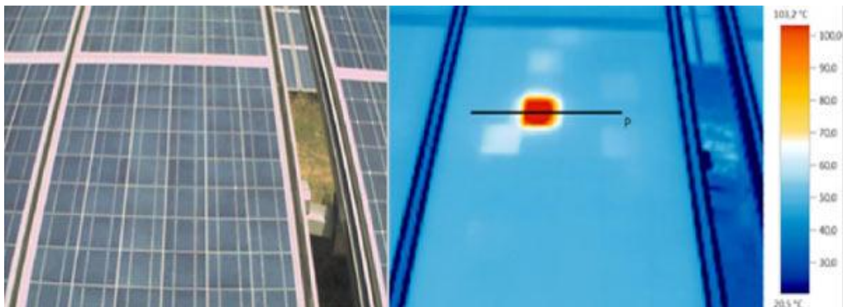
Obr. 3.2 Reálný snímek a termogram fotovoltaického modulu s vadnou buňkou. Na reálném snímku není žádná závada zjistitelná. [8]
