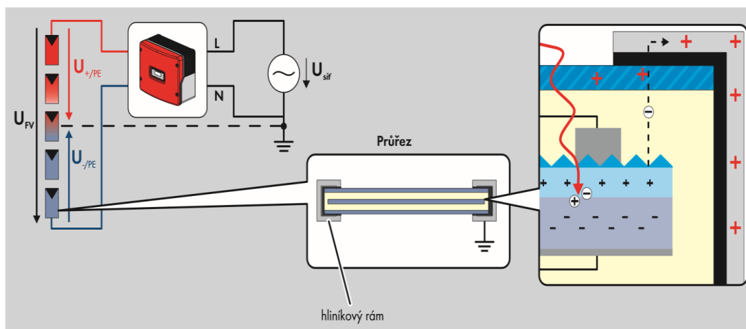
Obr. 4.1 Svodový proud je způsoben napěťovým potenciálem a způsobují jej negativní (-) ionty migrující od polovodičů a pozitivní (+), ionty migrující z obalu skla a vnějšího prostředí [11]
