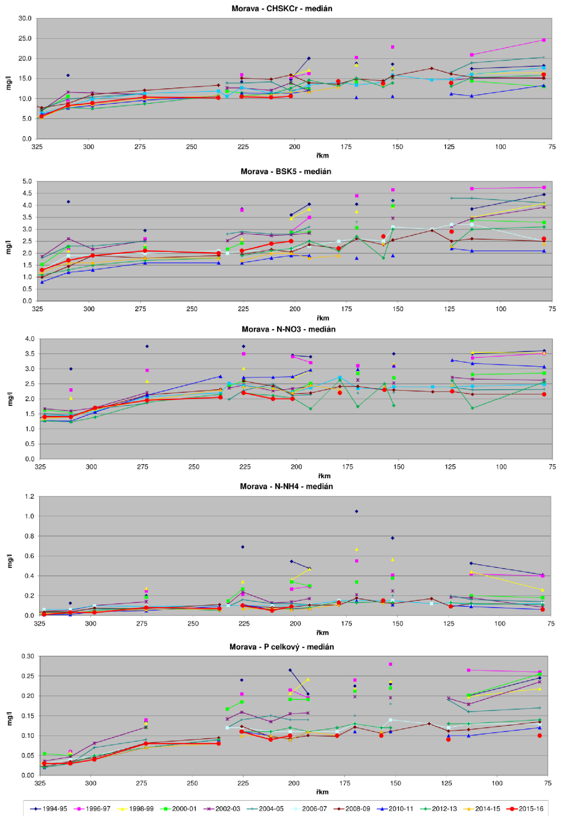
Obr. 3.6. Graficky zpracovaný podélný profil řeky Moravy v základních ukazatelích od roku 1994 do 2016 [18]
