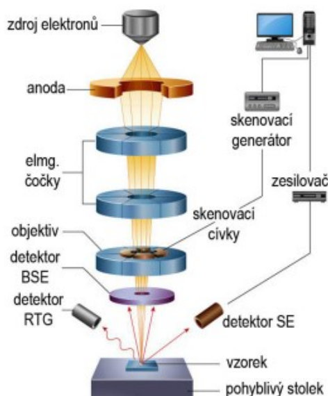
Obrázek 2.7: Schéma rastrovacího elektronového mikroskopu (Reichl a Všetická 2021)
