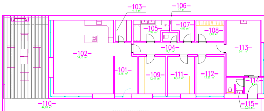
Obrázek 3 Dispozice rodinného domu
