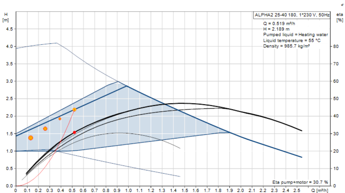
Obrázek 18 Průtoková charakteristika ALPHA2 25-40 [59]
