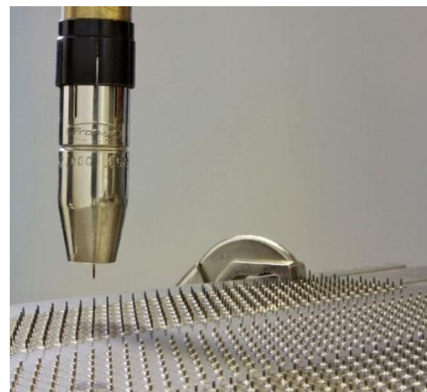
Obr. 35 CMT Pin [52].
