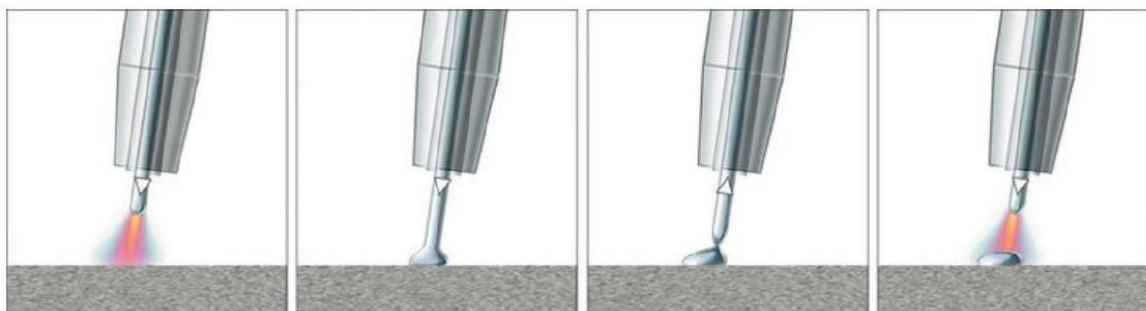
Obr. 32 Princip CMT [48].
