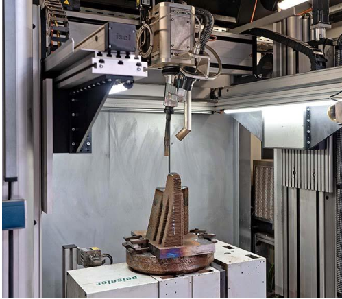
Obr. 18 CNC portál [25].
