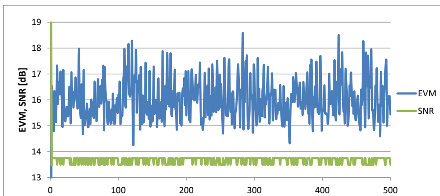
Obr. 7.11: Grafické znázornění odstupe signálu od šumu a velikosti odchylky vektoru pro jednotlivé pakety ve scénáři 1A.
