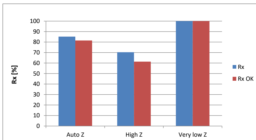
Obr. 7.5: Grafické znázornění správnosti doručení dat pro různá nastavení impedance.
