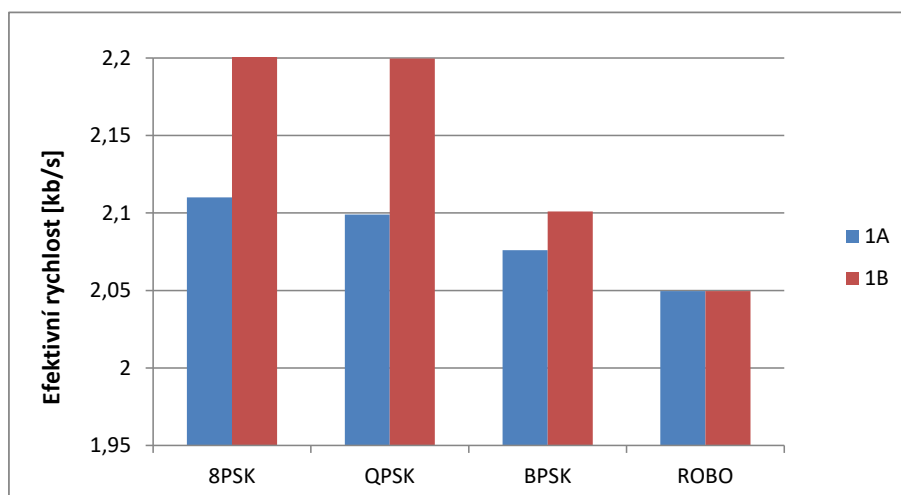
Obr. 7.1: Srovnání naměřené efektivní rychlosti pro scénář 1A a 1B.
