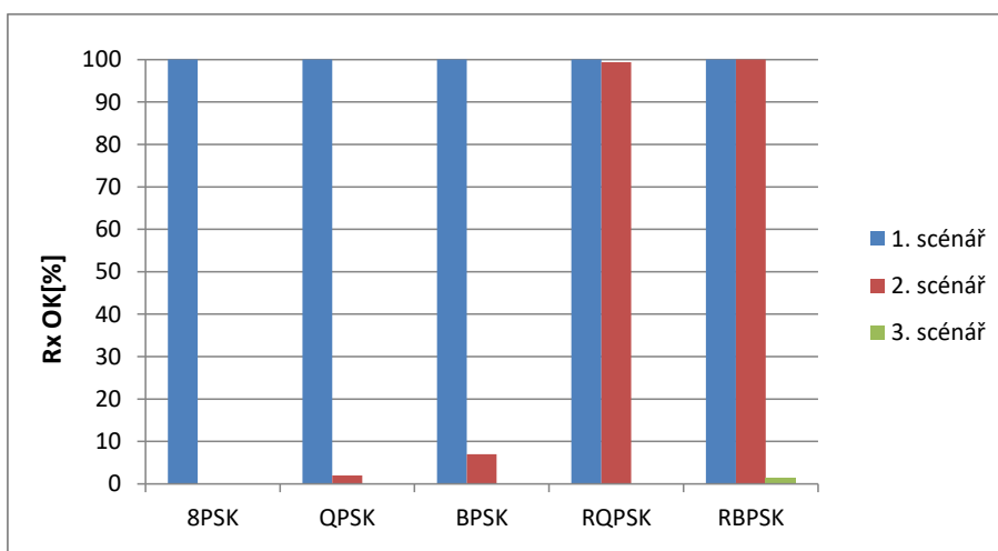
Obr. 7.10: Grafické znázornění správnosti doručených dat pro jednotlivé topologie dle užití modulační.
