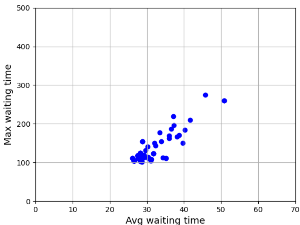
Obr 29: Vykreslení desáté generace odpolední dopravy genetického algoritmu.
