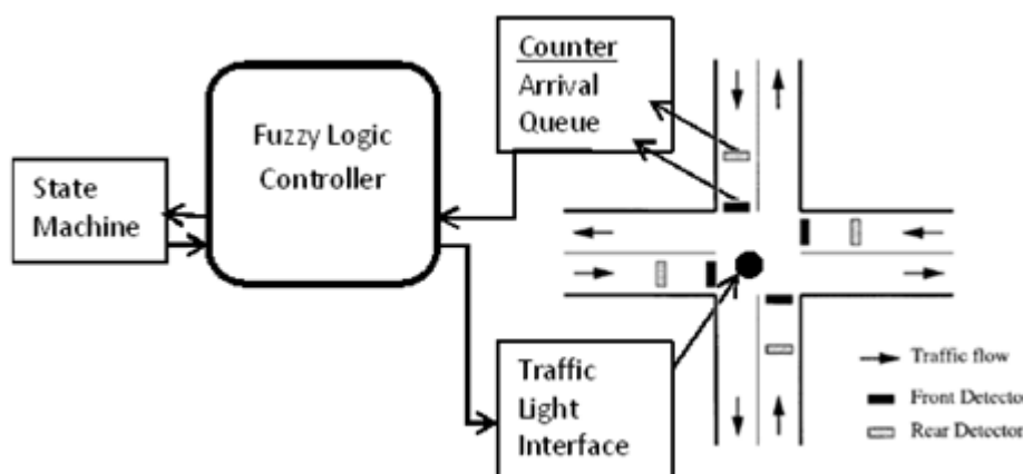
Obr. 4: Schéma fuzzy logiky využití k ovládní délky zelené fronty světelné křižovatky [15].
