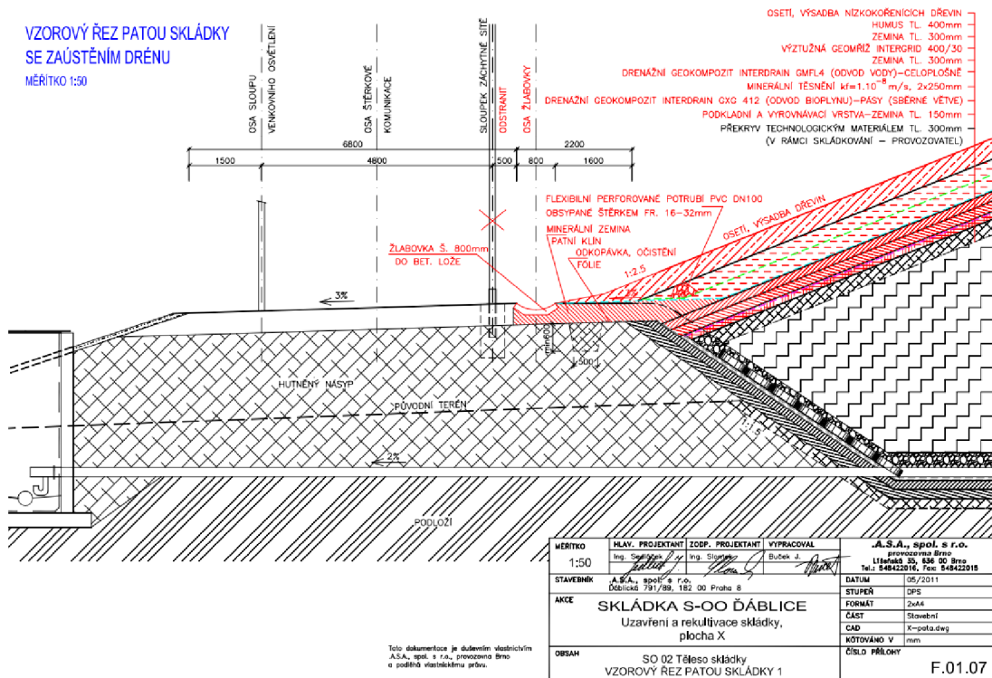
Obrázek 7: Vzorový řez patou skládky 1 (.A.S.A. spol. s r.o. 2011)
