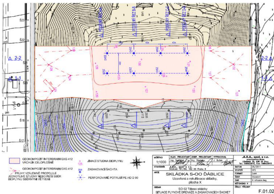
Obrázek 6: Situace plynové drenáže a zasakovacích šachet (.A.S.A. spol. s r.o. 2011)
