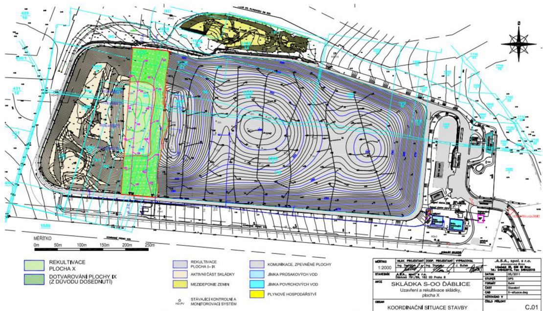
Obrázek 4: Koordinační situace stavby (.A.S.A. spol. s r.o. 2011)
