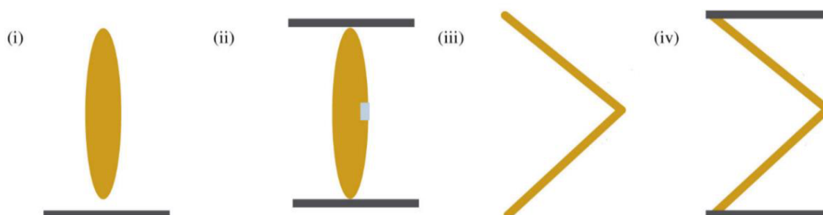
Obrázek 1: Je zde zobrazena geometrie separačního média (žlutá) a stěny (šedé) ukazují, zda je separační médium uzavřené nebo otevřené: označuje šedá barva a ploché nebo nálevkovité: žlutá barva (Hamann & Blake 2022).
