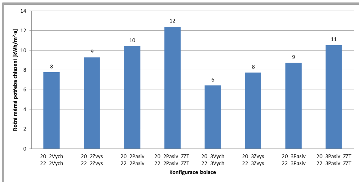
Obr. 5.18 – Roční měrná potřeba chlazení v závislosti na konfiguraci izolace vztahovaná na obytnou plochu dřevostavby.
