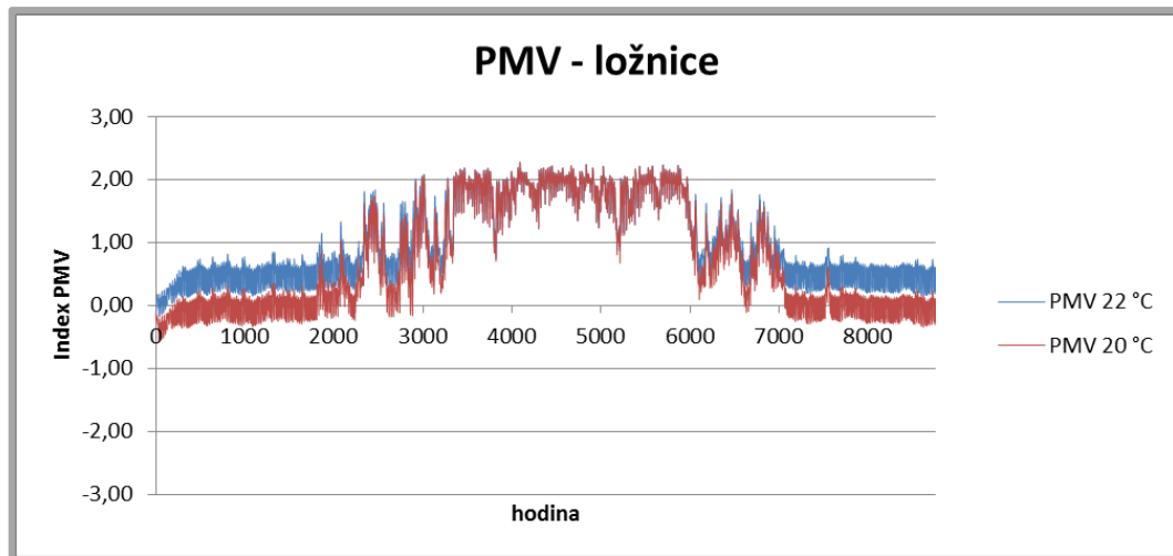
Obr. 5.23 - Index PMV ložnice 2.NP dřevostavby
