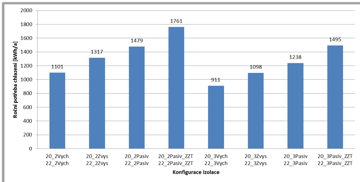
Obr. 5.17 – Roční potřeba chlazení v závislosti na konfiguraci izolace dřevostavby.
