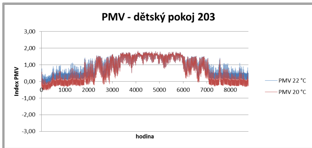
Obr. 5.24 - Index PMV dětského pokoje 203 2.NP dřevostavby
