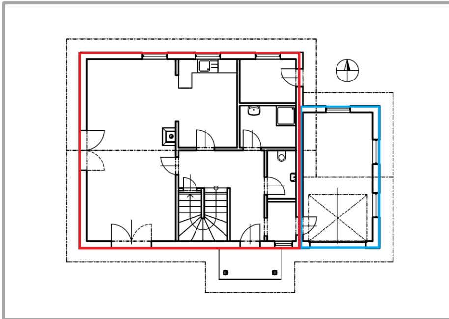
Obr. 3.5 – Půdorys 1.NP posuzované dřevostavby.
