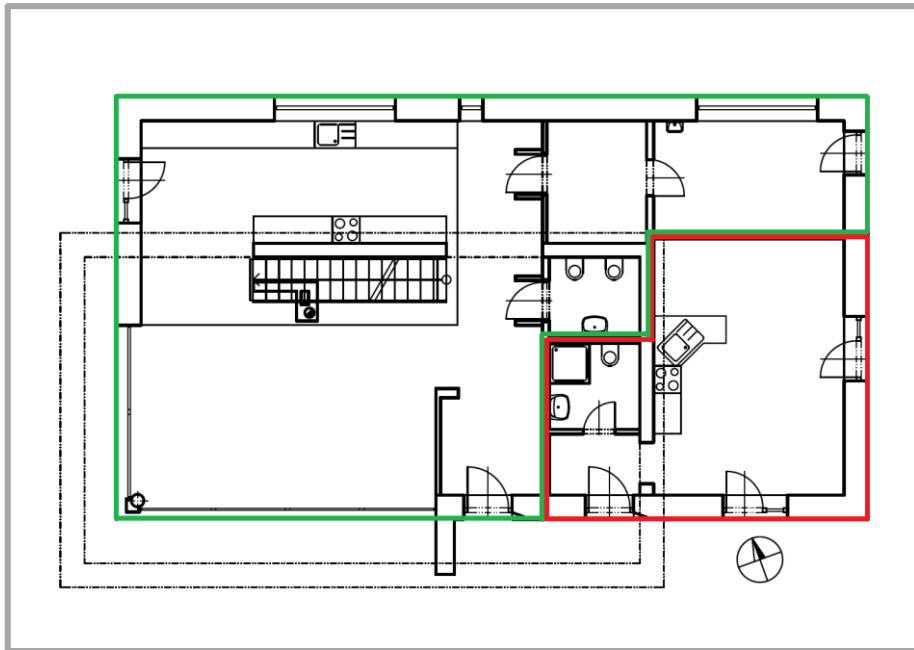
Obr. 3.2 – Půdorys 1.NP hodnocené zděné stavby.
