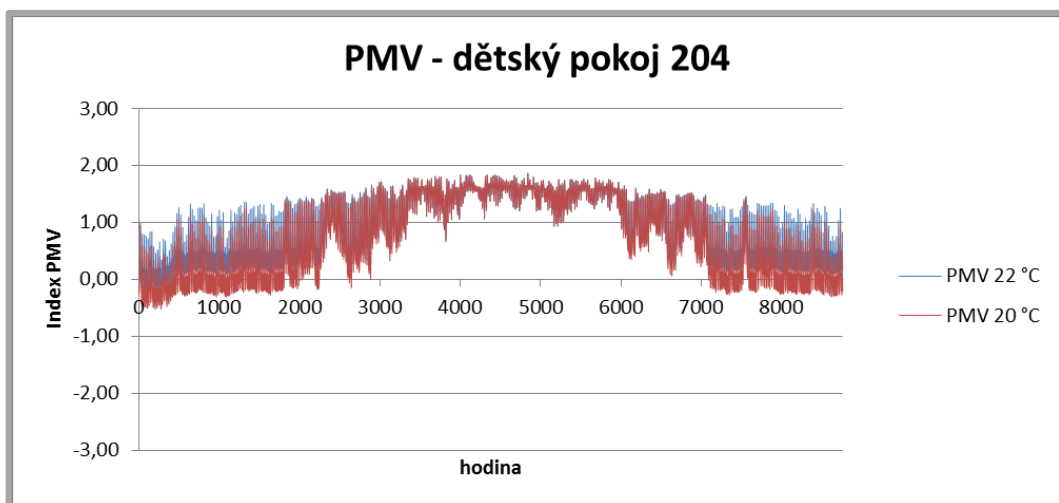
Obr. 5.25 - Index PMV dětského pokoje 204 2.NP dřevostavby
