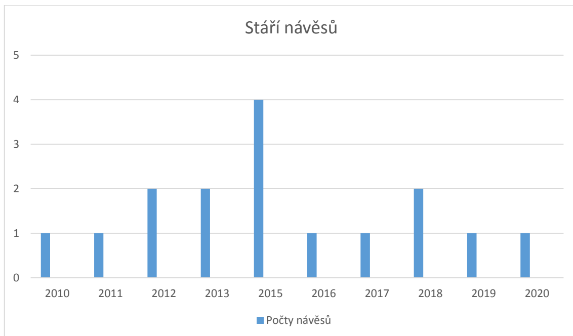
Obr. 2.5 Stáří návěsů
