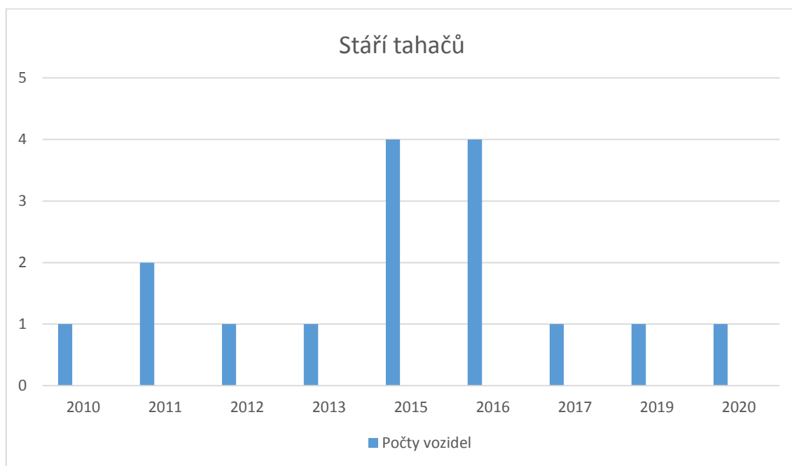
Obr. 2.4 Stáří tahačů
