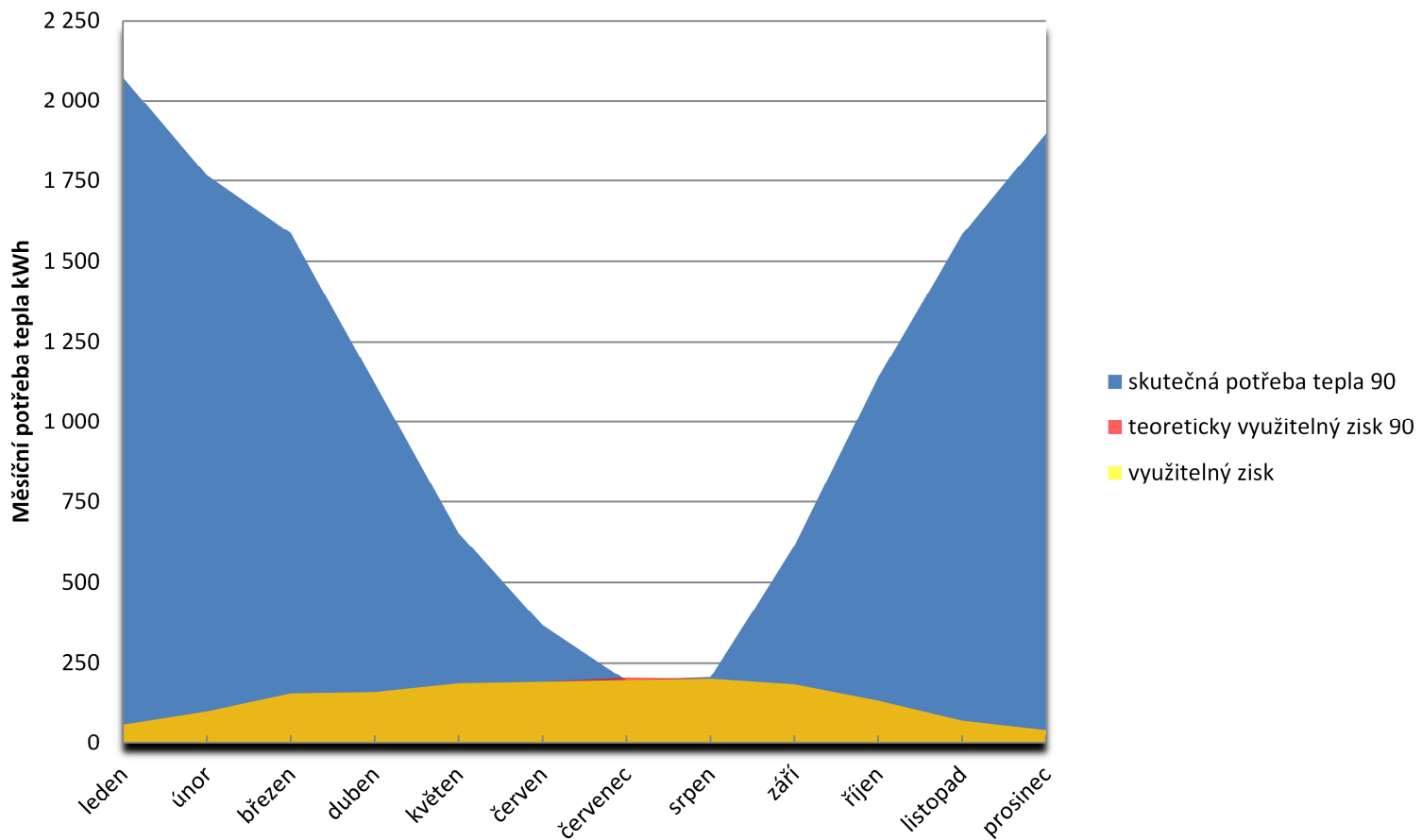
Graf B-10 : Celkové pokrytí potřeby tepla při úhlu 90°
