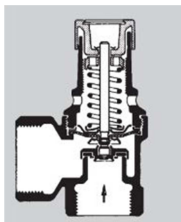
Obr. B-4 : Pojistný ventil Honeywell SM 120-Z [8]
