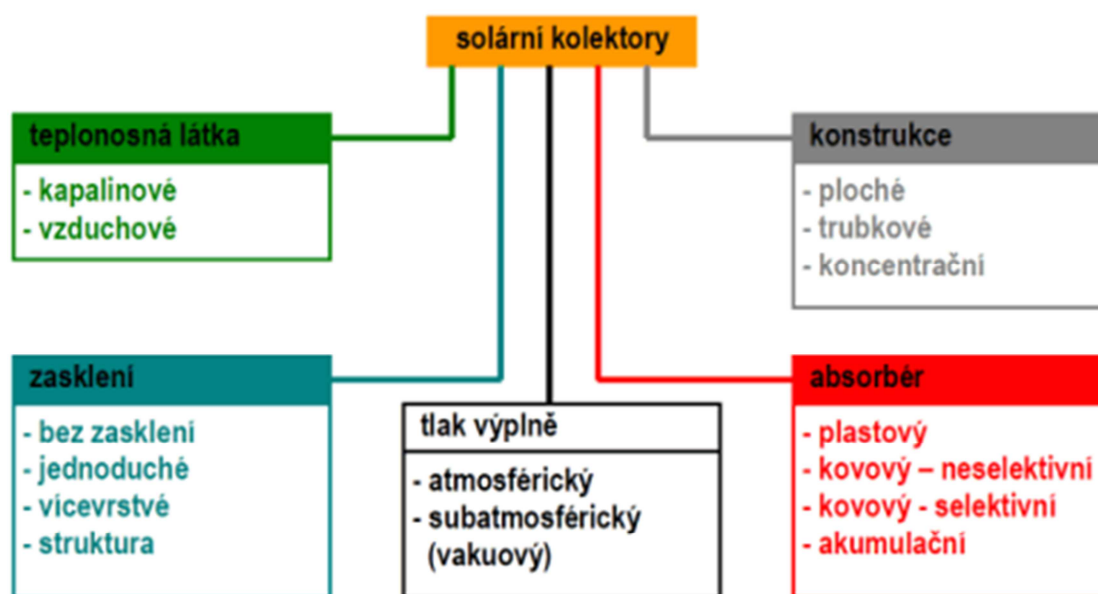
Obr. A-5 : Rozdělení termických kolektorů [3]
