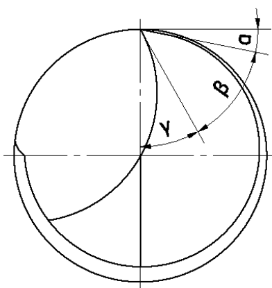
α- úhel hřbetu, β- úhel břitu, γ- úhel čela
