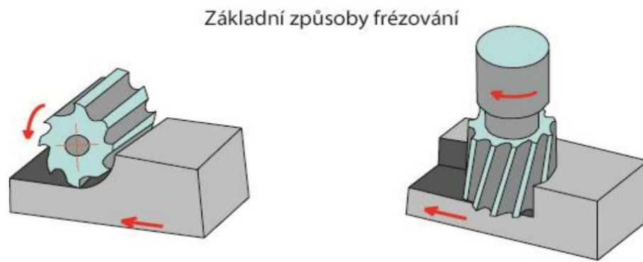
Obr. 2- Plošné a čelní frézování[3]
