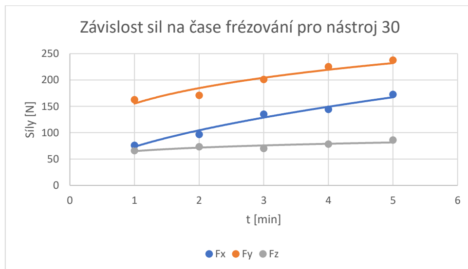
Graf 9. Závislost sil na čase pro nástroj Gama 30^\circ s ochranným povlakem ALOX SN 2
