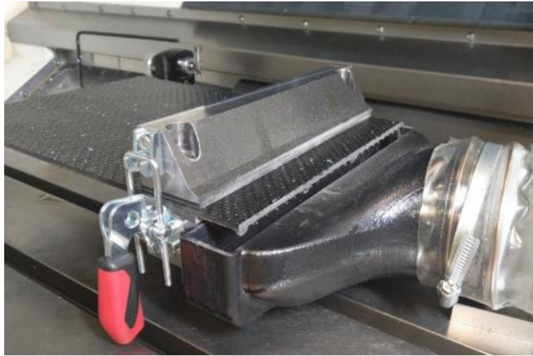
Obr. 29- Upínací přípravek [28]
