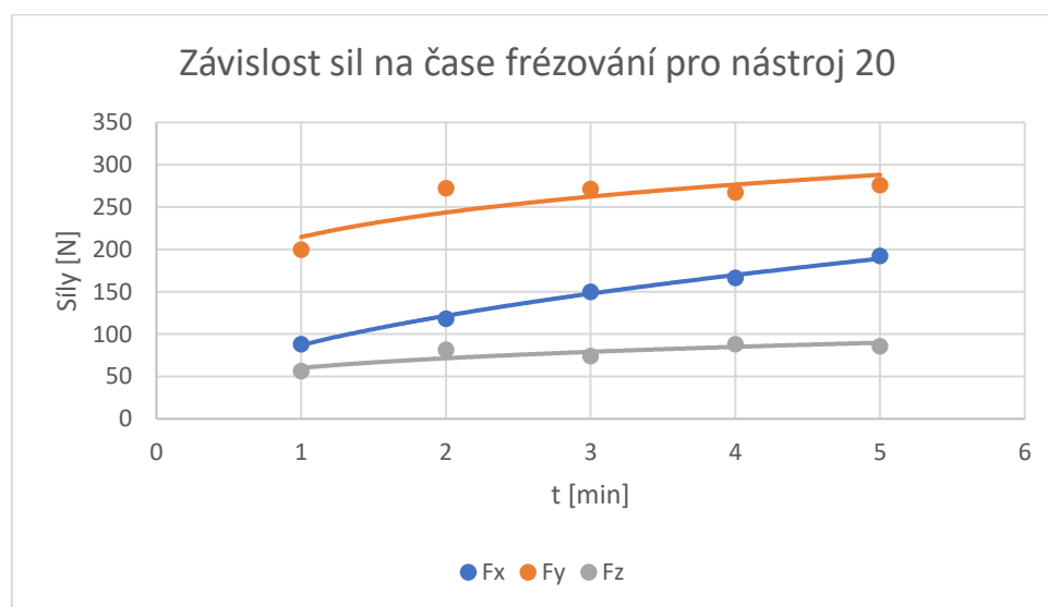
Graf 8. Závislost sil na čase pro nástroj Gama 20^\circ s ochranným povlakem ALOX SN 2
