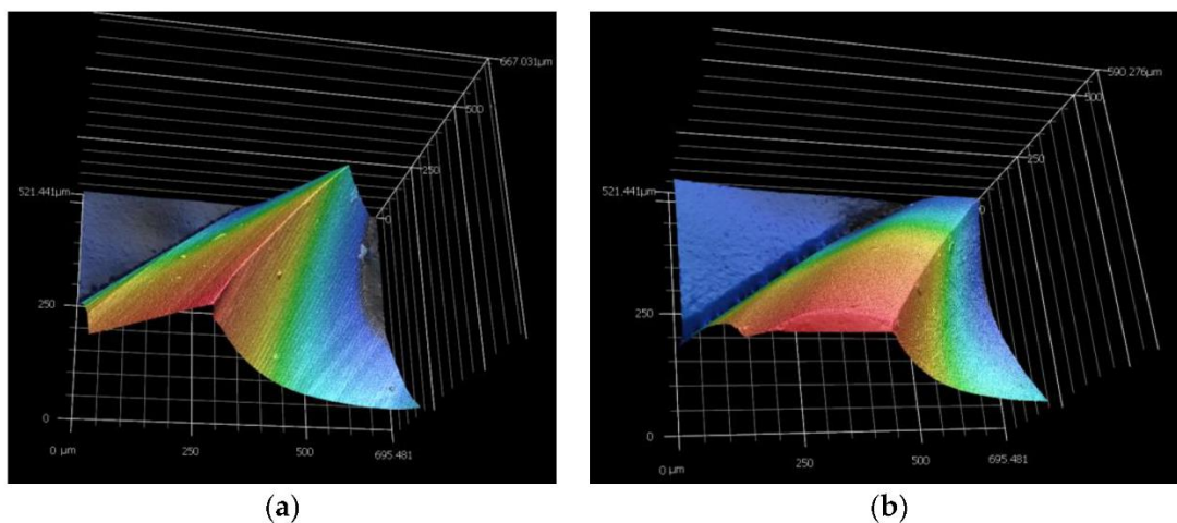
Obr. 7- Detail ostří nástroje: a) nové ostří; b) opotřebované ostří[13]
