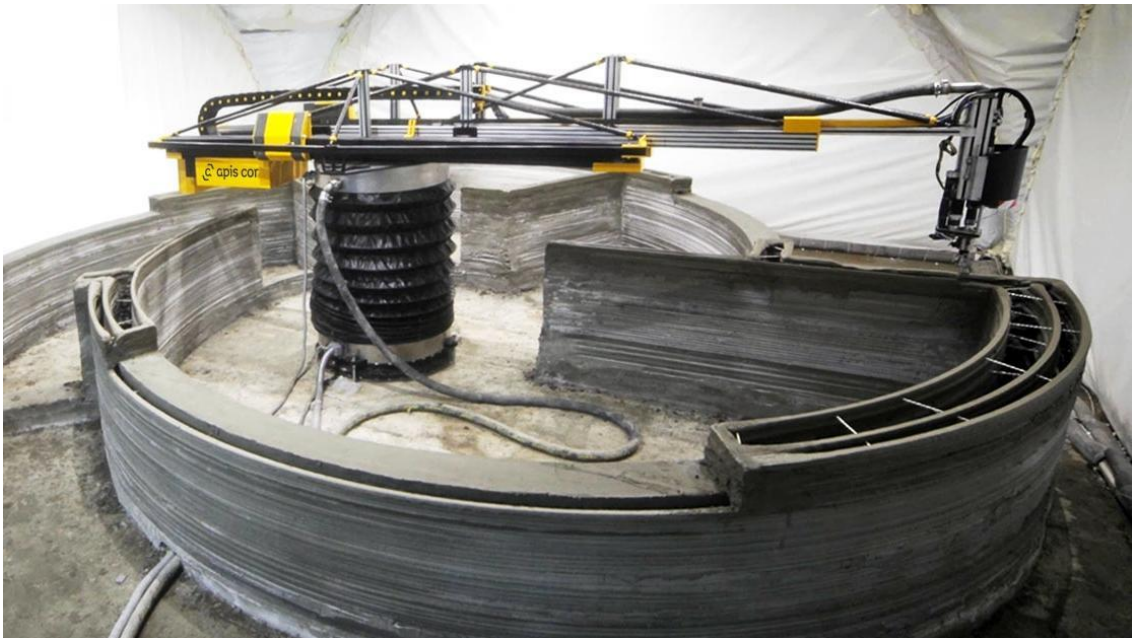
Obr. 1 Průběh tisku domu pomocí jednoramenné 3D tiskárny [10].
