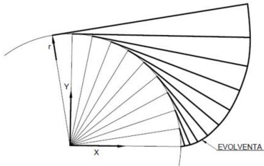
Obr. 18 Evolventní tvar boku zubu (prostá evolventa) [27].
