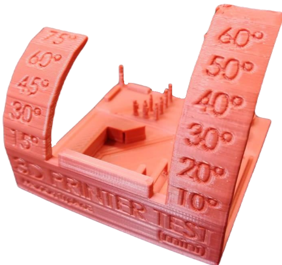
Obr. 48 Test filamentu.
