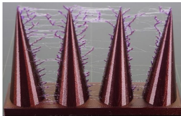
Obr. 5 Nežádané odkapávání filamentu během tisku [21].
