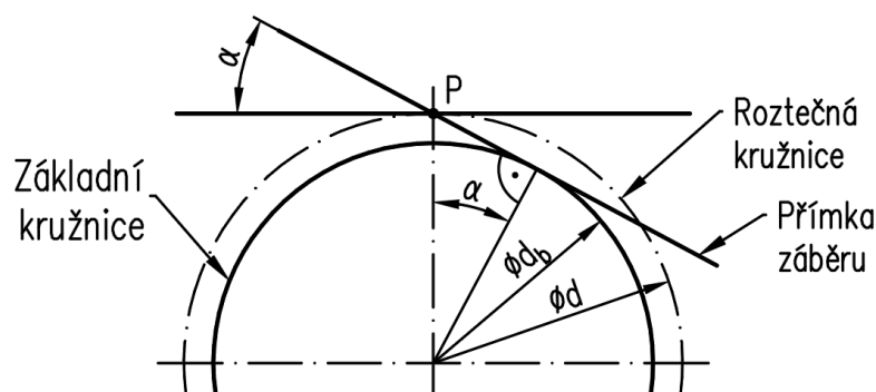
Obr. 20 Úhel záběru [45].
