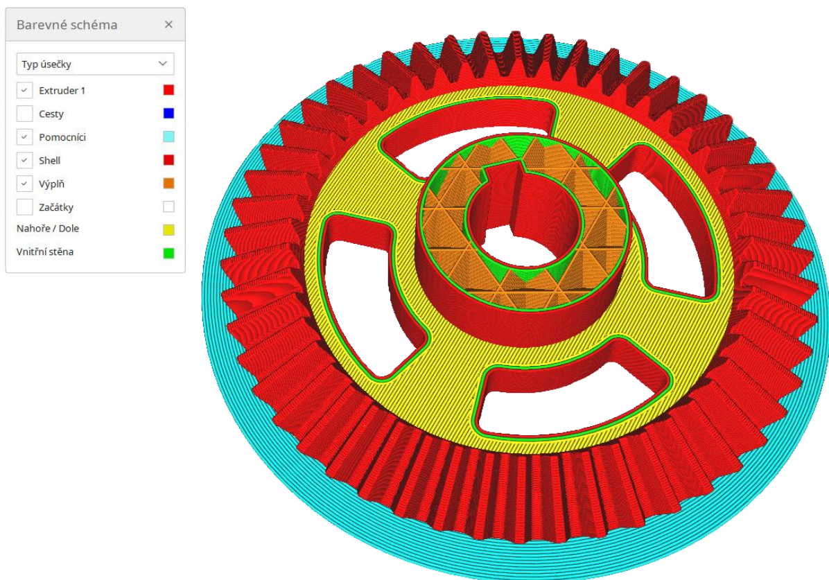
Obr. 49 Zobrazení průběhu tisku na kuželovém ozubeném kolu hnaném.
