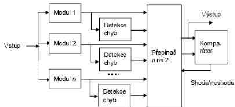
Obrázek 2.16 Systém se zálohovanou dvojicí
