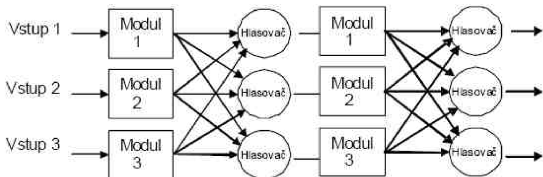
Obrázek 2.12 Vícestupňový TMR
