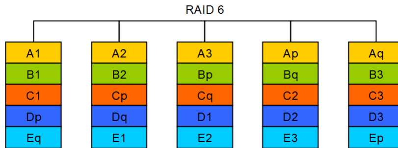
Obr. 6.7: Schéma zapojení diskového pole RAID 6
