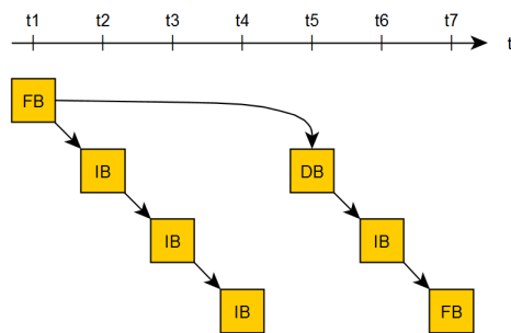
Obr. 2.4: Schéma kombinované zálohy
