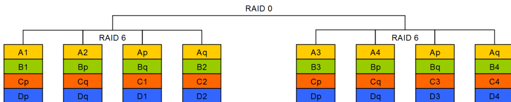
Obr. 6.10: Schéma zapojení diskového pole RAID 60
