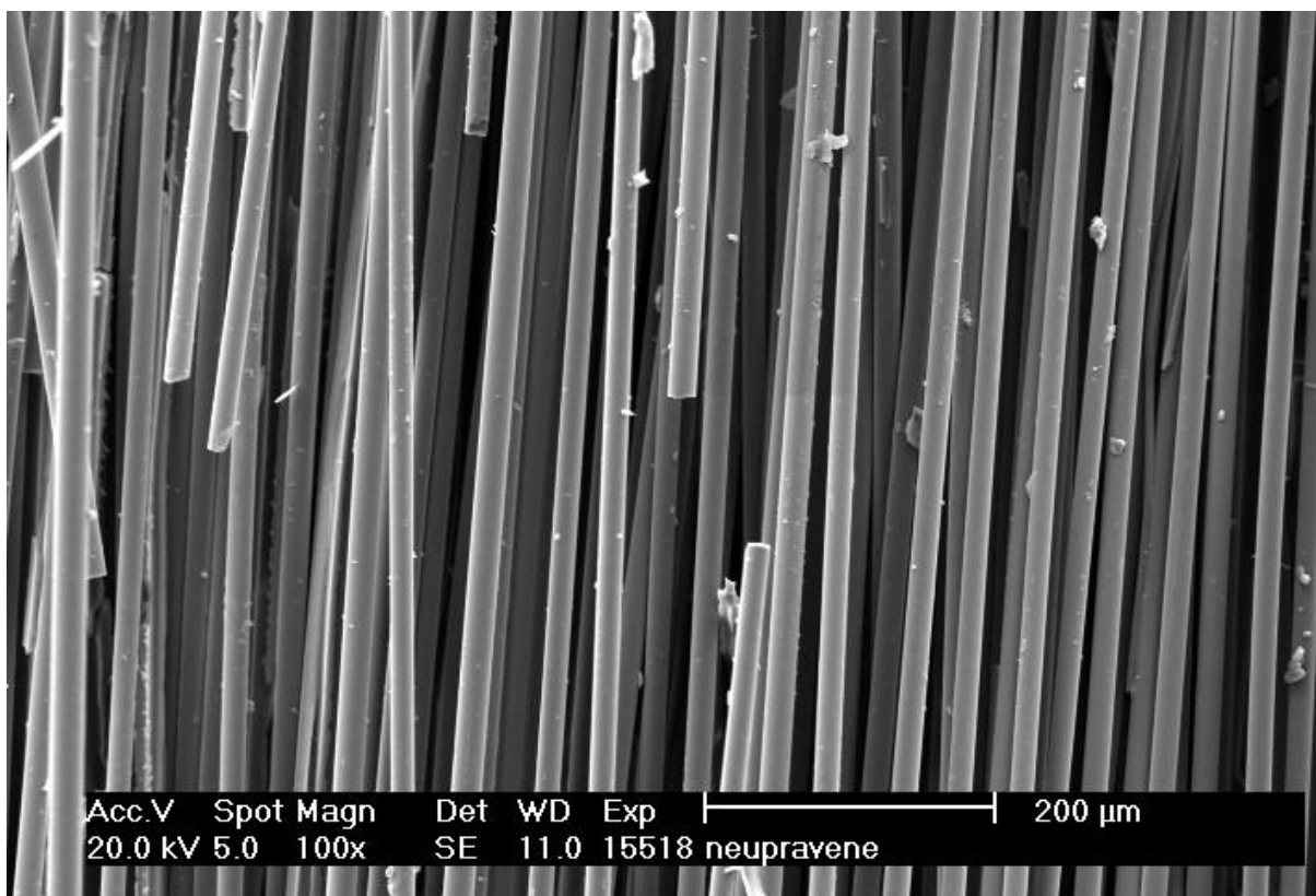
Obr. 4.19: Snímek SEM porušeného kompozitu s neupravenými vlákny
