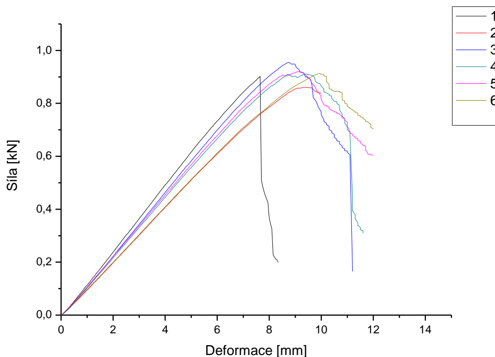
Obr. 4.10: Graf závislosti průhybu vzorku na působící síle: upravená vlákna, V_f = 40\%
