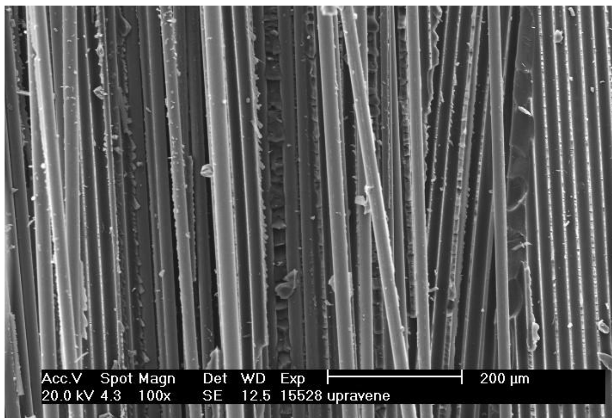
Obr. 4.20: Snímek SEM porušeného kompozitu s upravenými vlákny
