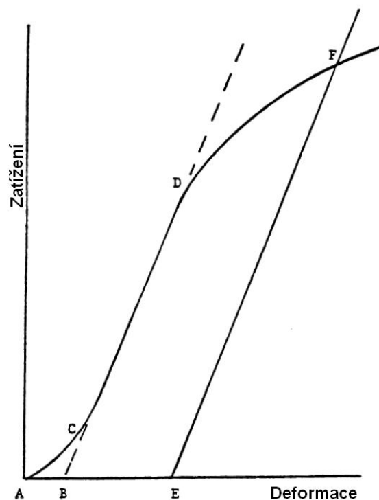
Obr. 3.8: Schematický graf závislosti průhybu na zatížení s oblastí elastické deformace (upraveno)
