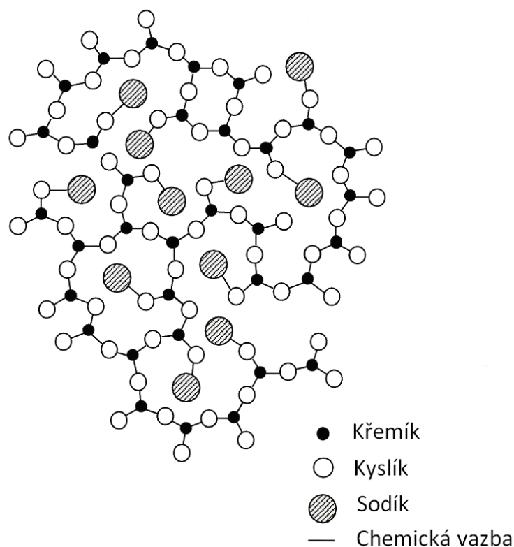
Obr. 2.4: Model amorfnní atomární struktury skla (upraveno) [13]
