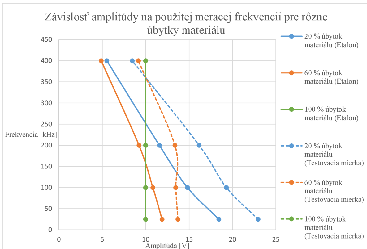
Obr. 6.4 Závislosť amplitúdy signálu na použitej meracej frekvencii
