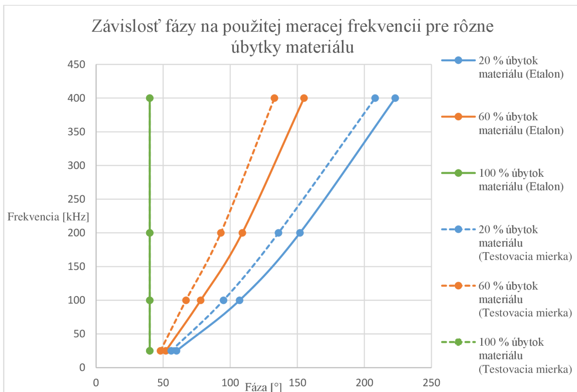
Obr. 6.5 Závislosť fázy signálu na použitej meracej frekvencii
