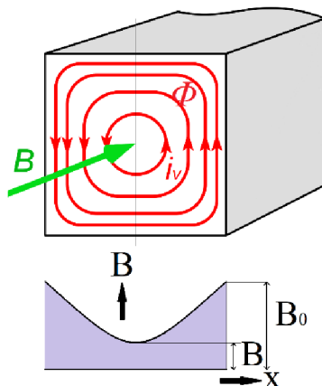
Obr. 4.2 Zobrazenie účinkov povrchového javu [14]
