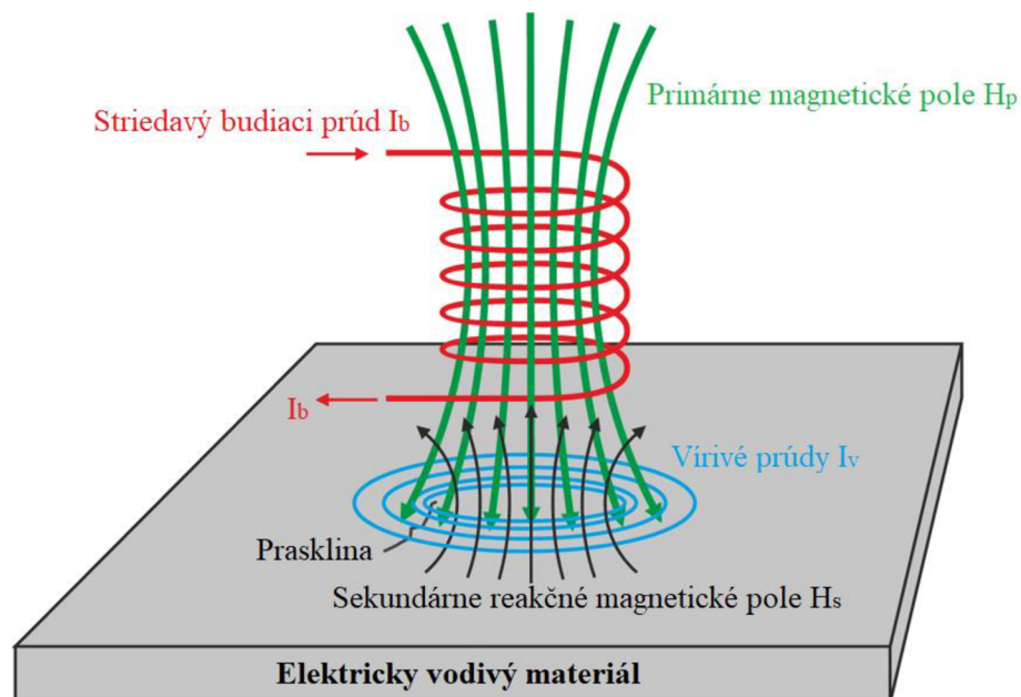
Obr. 4.5 Princíp priložnej cievky [13]
