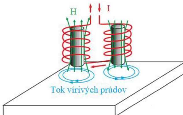
Obr. 4.3 Princíp diferenciálneho zapojenia cievok v samo-porovnávacom režime [13]
