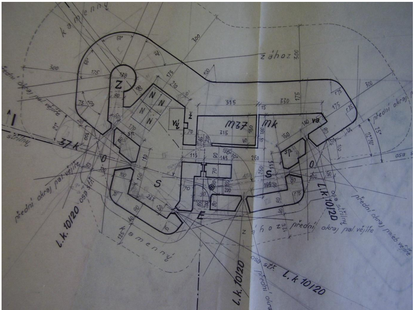
Obr. 15 – příklad projekce pěchotního srubu – rozvržení výbroje a vybavení v horním patře objektu RS – 89, archiv J. Hrubického
