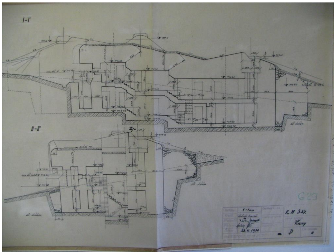
Obr. 13 – příklad projekce pěchotního srubu – podrobný řez srubem KS – 37, archiv J. Hrubeckého
