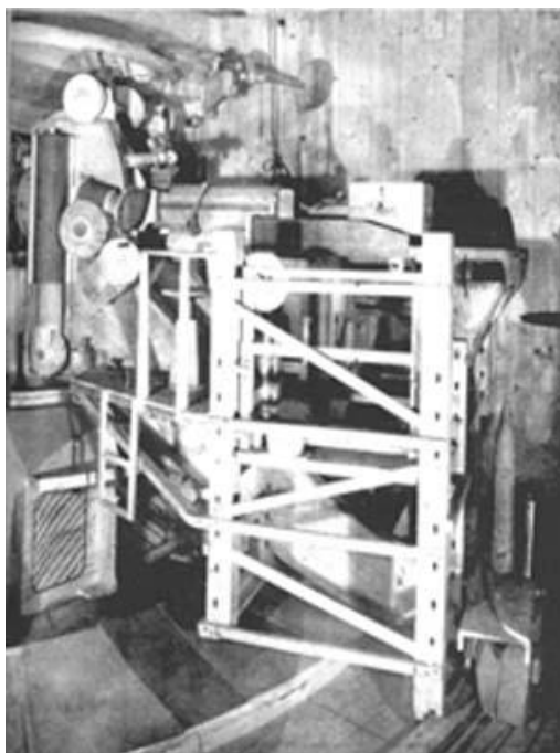
Obr. 123 – tovární dřevěný model houfnice vz. 38 ve Škodových závodech v Plzni, 1938, archiv J. Hrubeckého
