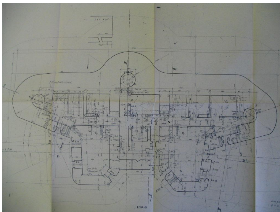
Obr. 14 – příklad projekce pěchotního srubu – podrobný půdorys objektu KS – 37, archiv J. Hrubeckého
