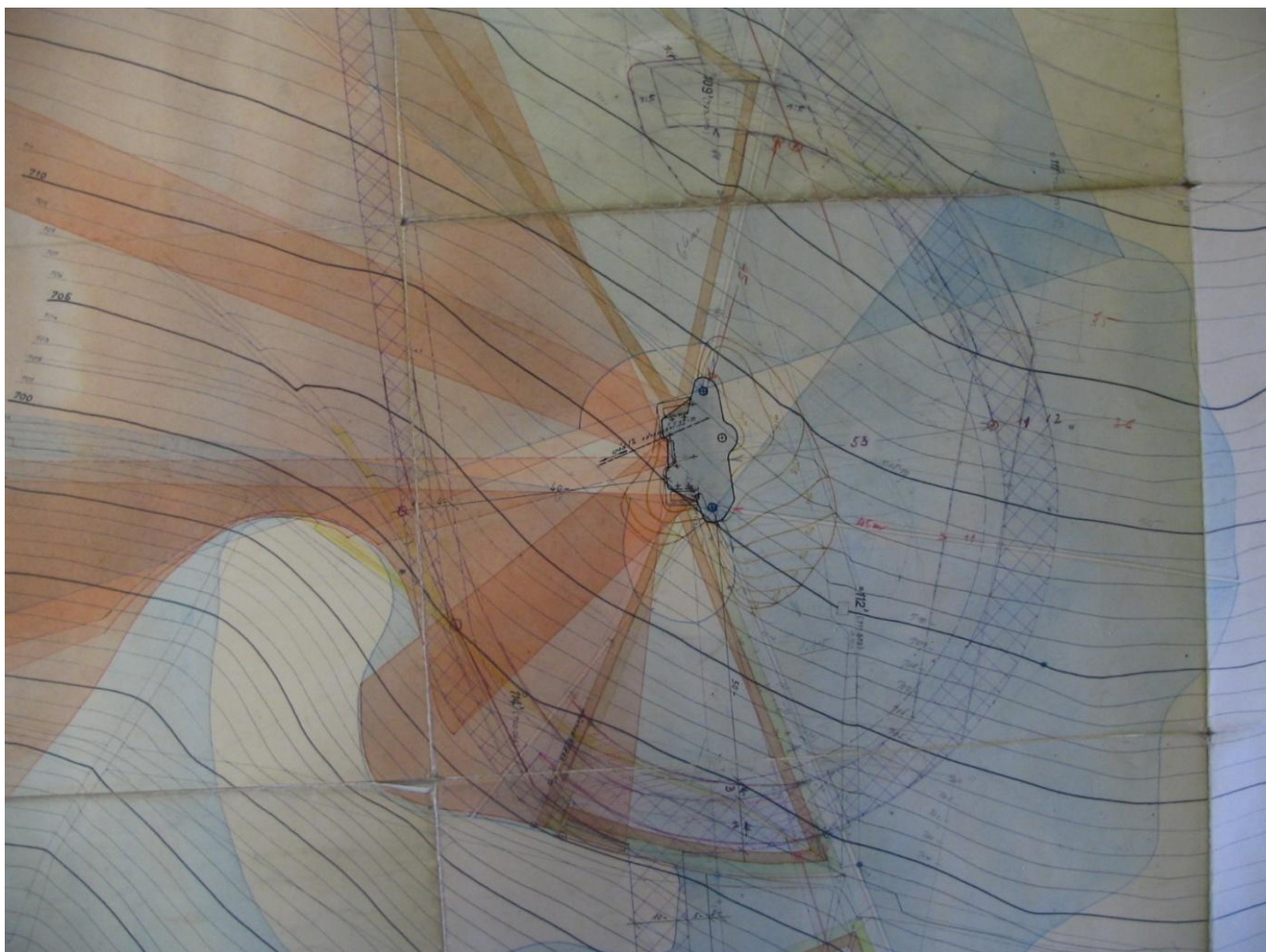
Obr. 12 – příklad projekce pěchotního srubu – plán překážkového systému a palebných vějířů srubu KS – 37, archiv J. Hrubeckého
