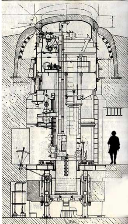
Obr. 124 – schematický náčrt otočné a výsuvné věže F3V, archiv J. Hrubeckého
