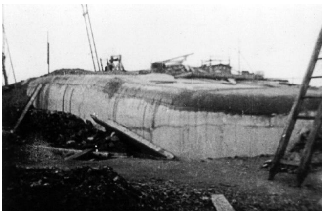
Obr. 122 – objekt pro otočnou a výsuvnou věž pro dvojče houfnice vz. 38 ráže 100 mm, zde měl za květnové částečné mobilizace v r. 1938 velitelské stanoviště pplk. Kostrhún, září 1938, archiv J. Hrubeckého
