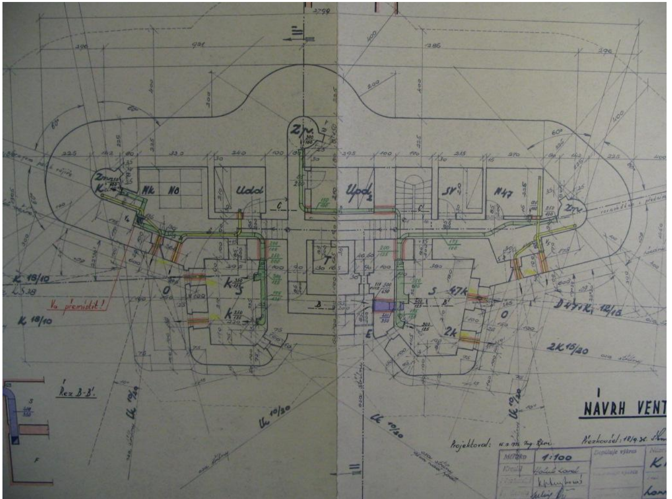
Obr. 11 – příklad projekce pěchotního srubu - plán filtroventilačního systému ve srubu KS – 37, archiv J. Hrubeckého
