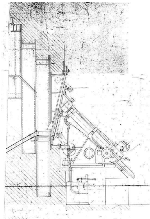
Obr. 125 – schematický náčrt zobrazující minomet vz. 38 ráže 90 mm a střílnu pro palbu z dolního patra pěchotního srubu, archiv J. Hrubeckého
