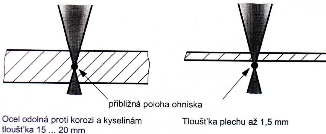
Obr. 4.3 Plazmové řezání (10)
