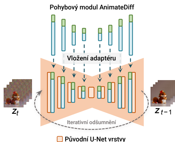
Obrázek 2.9: Princip pohybového adaptéru AnimateDiff
