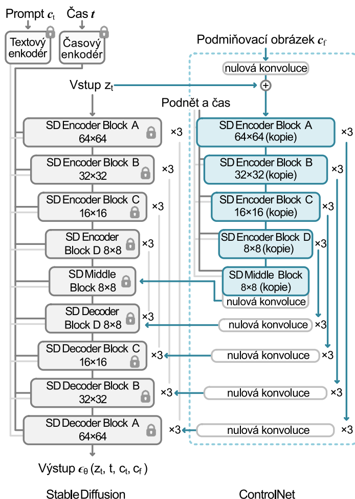
Obrázek 2.7: Schéma architektury ControlNet. Převzato z [28] (Upraveno).
