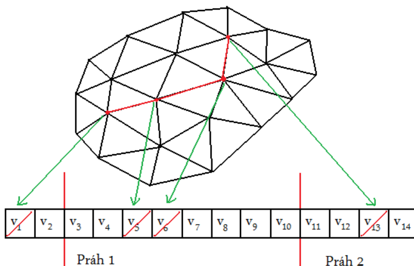
Obrázek 2.4.1 – Popis algoritmu
