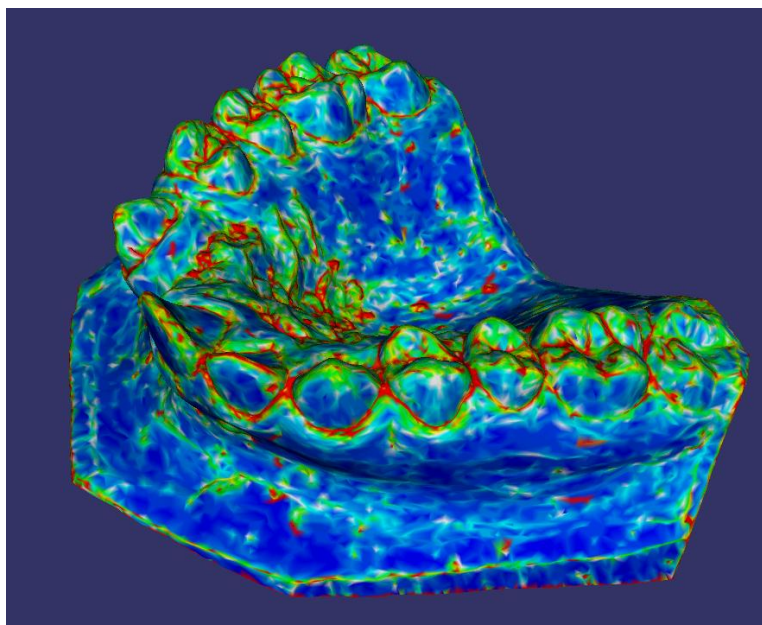
Obrázek 4.1.1 – Střední křivost
