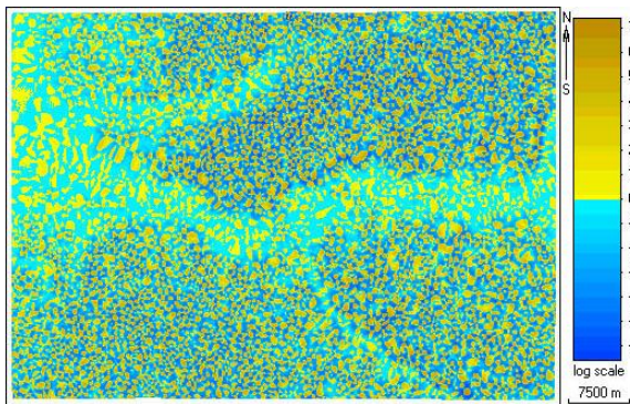
Obrázek 1.3.4 – Gaussova křivost
