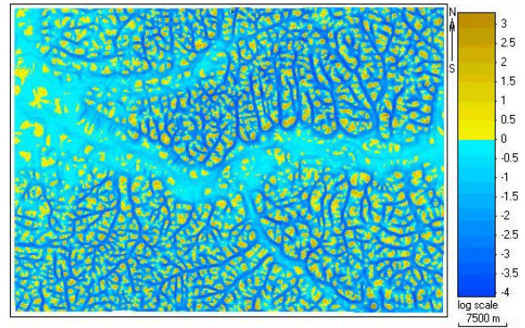
Obrázek 1.3.3 – Minimální křivost
