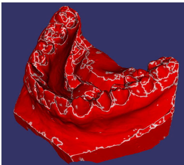
Obrázek 4.1.4 – Model 2, Watershed
