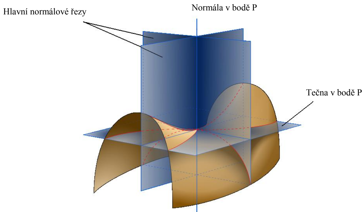
Obrázek 1.3.1 – Hlavní křivosti [7]
