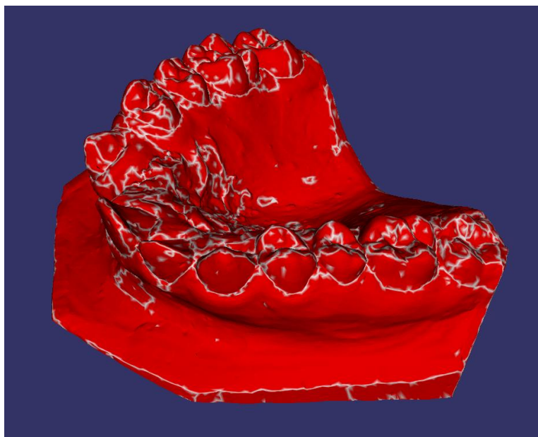
Obrázek 4.1.3 – Model 1, Watershed
