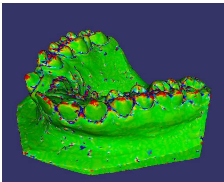
Obrázek 4.1.2 – Gaussova křivost
