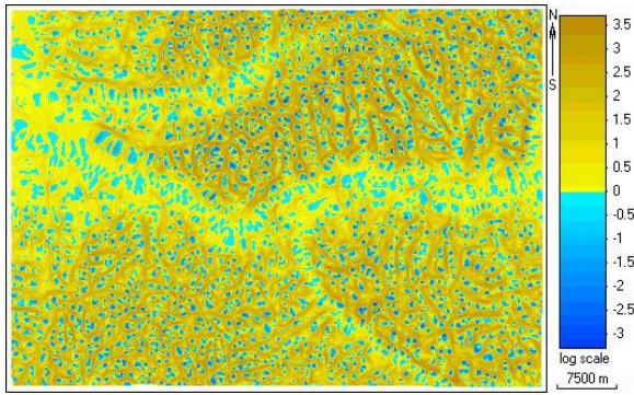
Obrázek 1.3.2 – Maximální křivost
