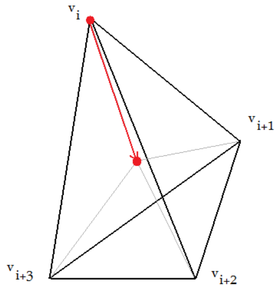
Obrázek 1.4.1 – Laplaceovo vyhlazení
