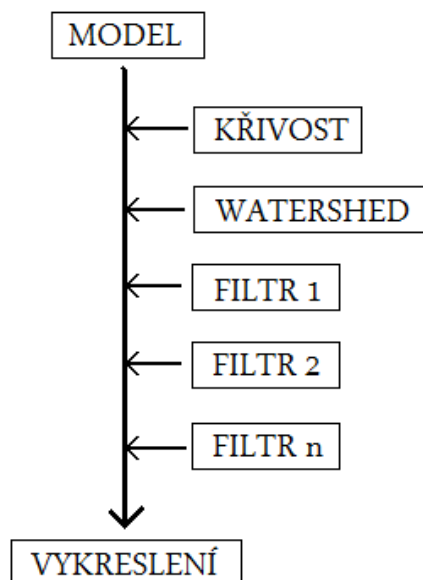
Obrázek 2.5.7 – Návrh aplikace
