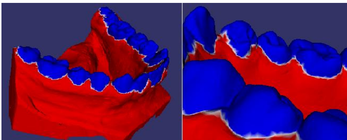
Obrázek 4.1.6 – Model 2, autodetekce
