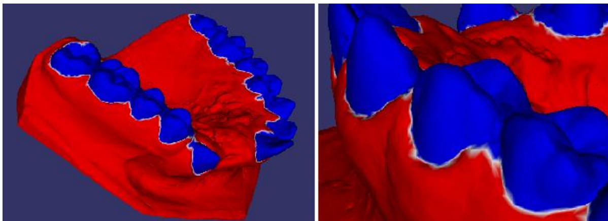
Obrázek 4.1.5 – Model 1, autodetekce
