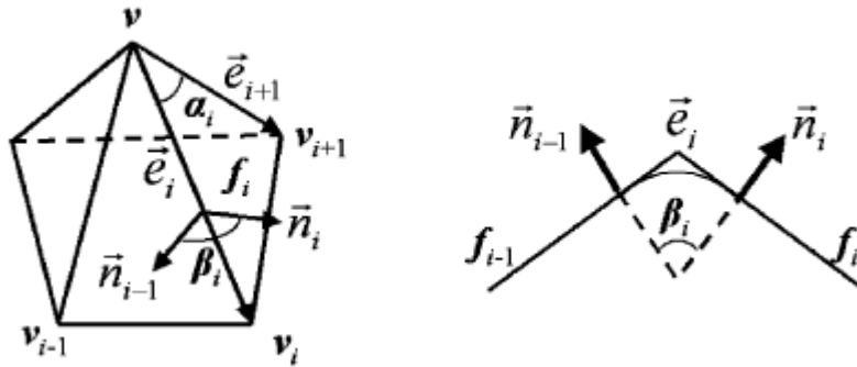
Obrázek 2.3.1 – Popis modelu
