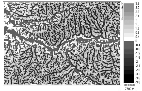
Obrázek 1.3.5 – Střední křivost
