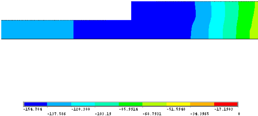
Obr. 39 Rozložení tlaků v blízkosti změny průřezu VAR56
