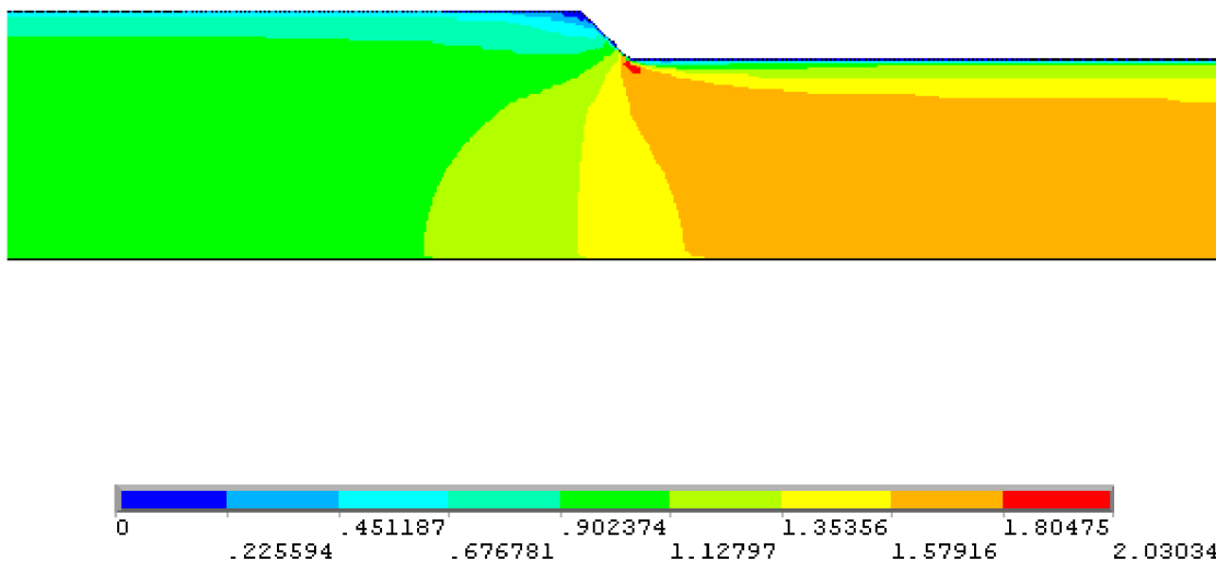
Obr. 40 Rozložení rychlostí v blízkosti změny průřezu VAR66
