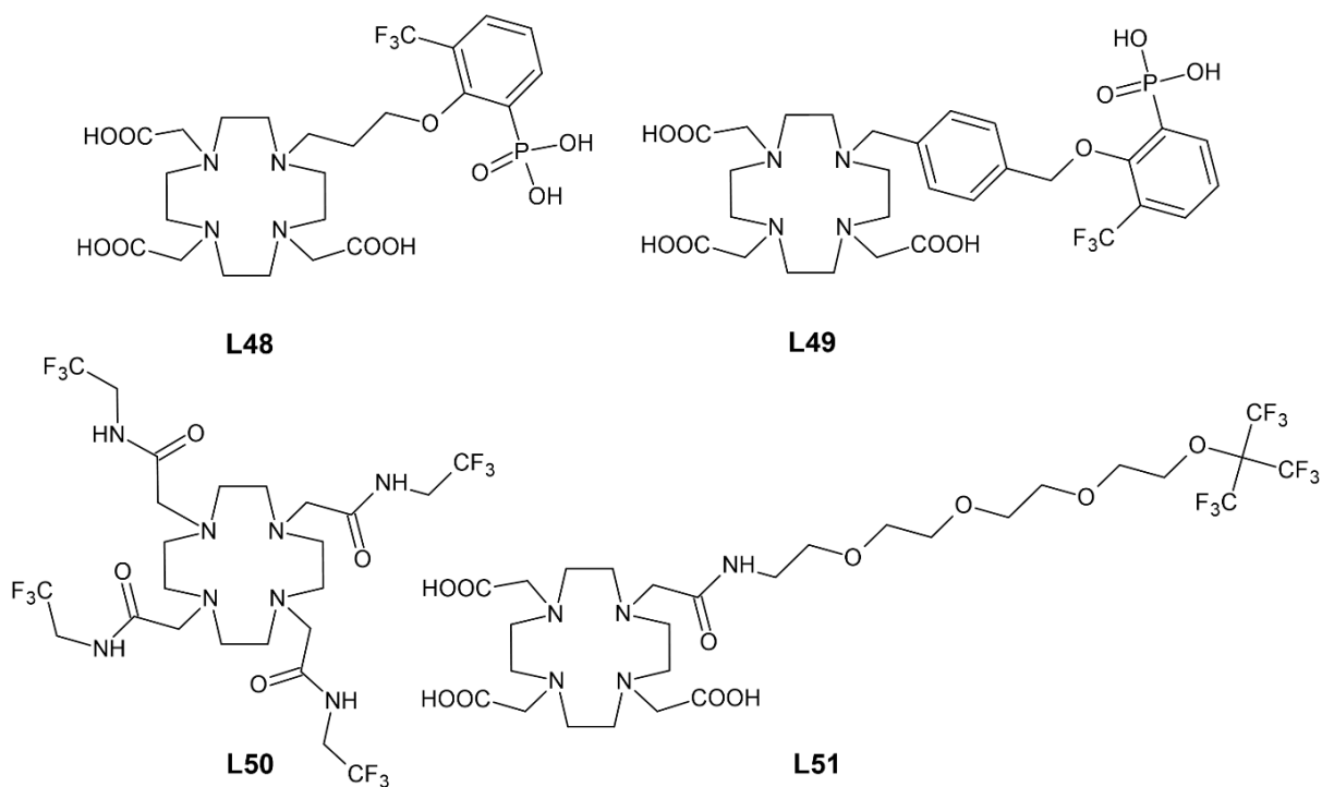
Obrázek 6 Strukturní vzorce ligandů L48–L51
