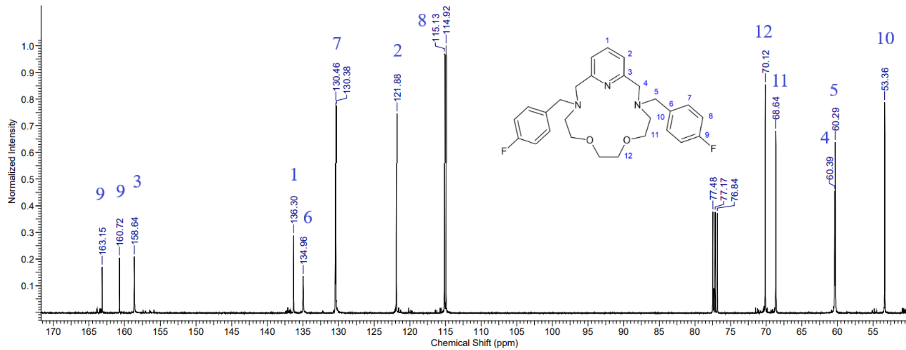
Obrázek 22 Naměřené 13 C NMR spektrum ligandu M2
