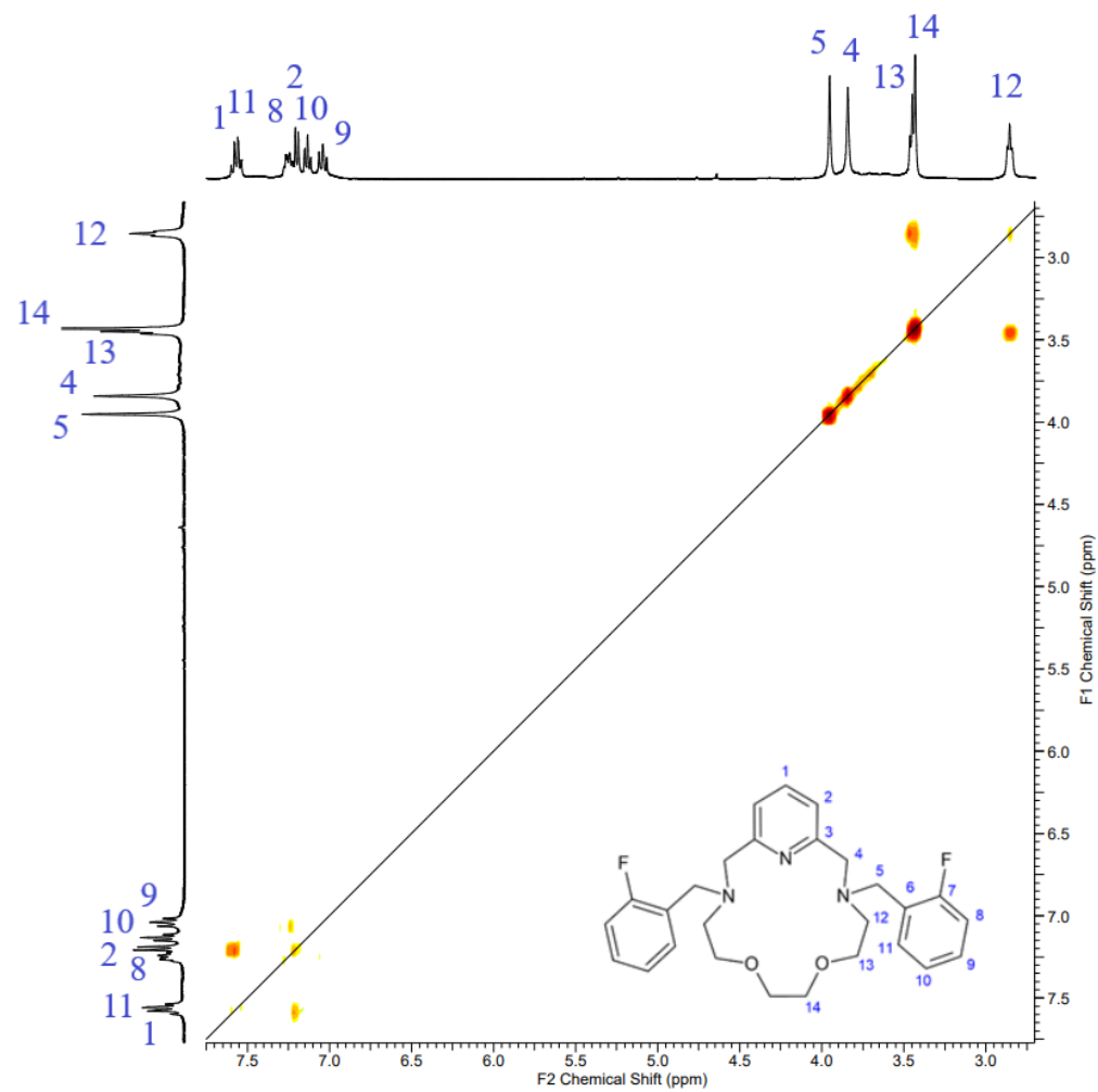
Obrázek 36 Naměřené ^1\text{H} - ^1\text{H} gs-COSY spektrum ligandu M4
