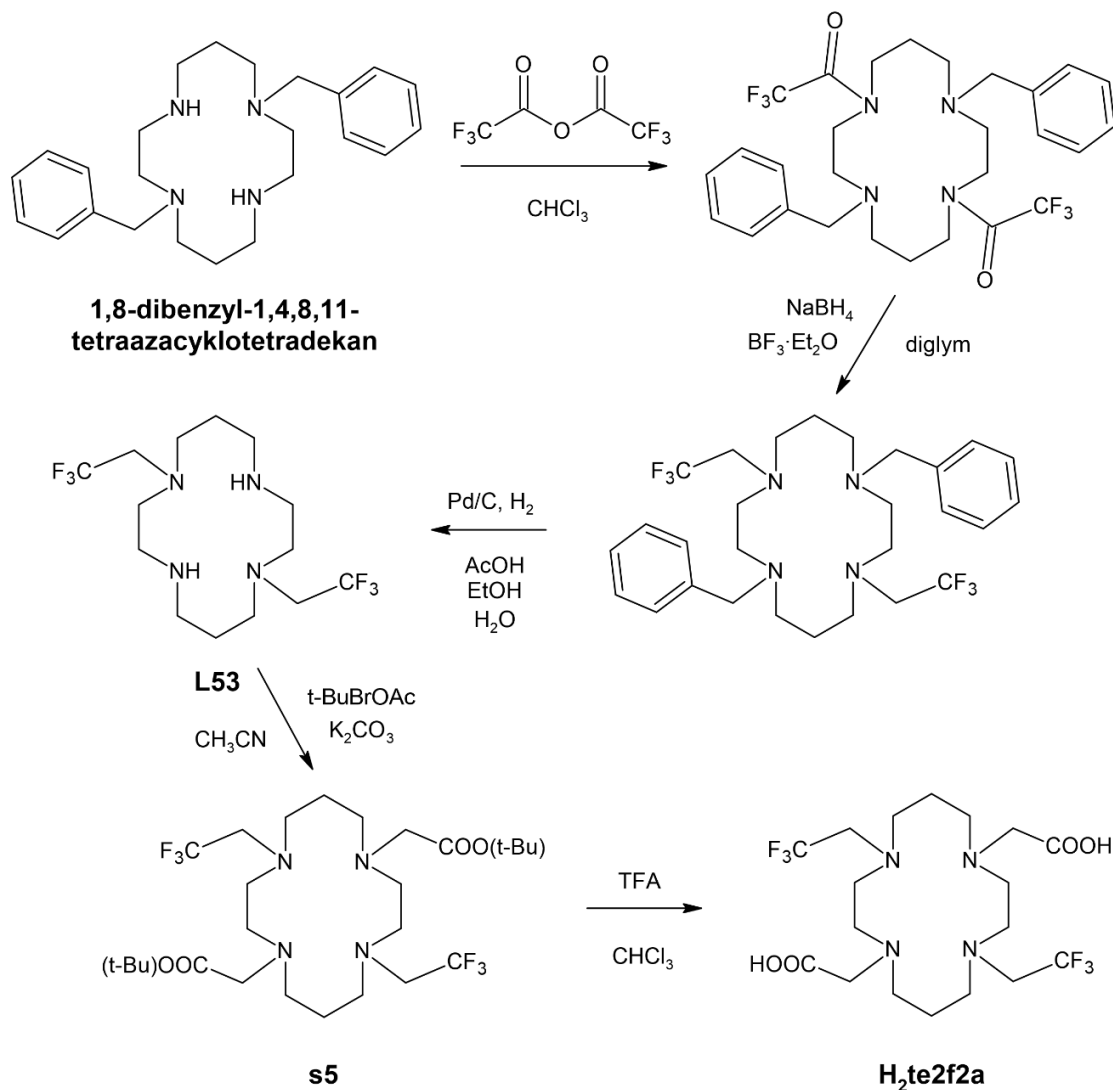
Obrázek 11 Reakční schéma přípravy H 2 te2f2a podle literatury. (46, 47)
