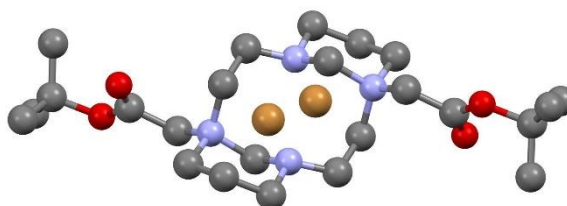
Obrázek 13 Molekulová struktura s3 získaná pomocí rentgenové strukturní analýzy. Atomy vodíku jsou pro přehlednost vynechány. Barvy atomů: uhlík – šedá; dusík – světle modrá; kyslík – červená; brom – oranžová.
