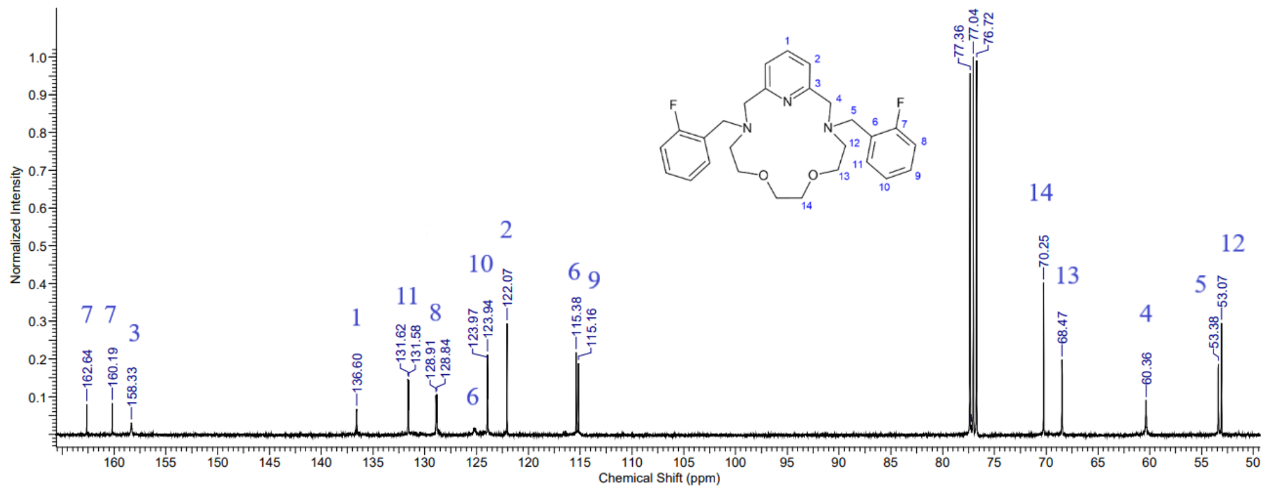
Obrázek 34 Naměřené 13 C NMR spektrum ligandu M4
