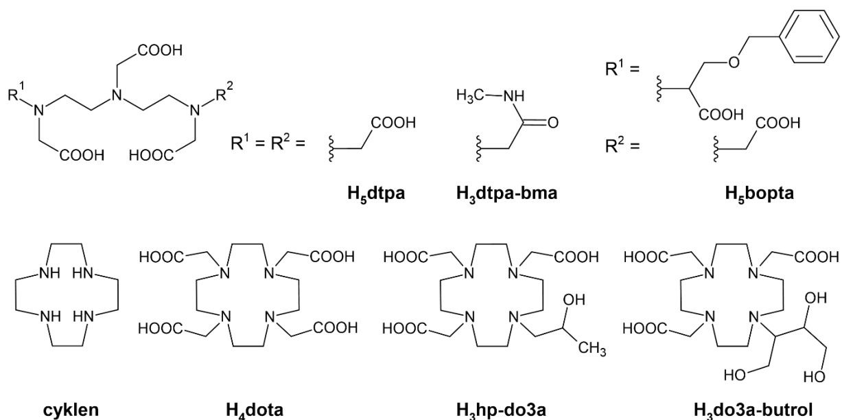
Obrázek 3 Strukturální vzorce necyklických i makrocyclických ligandů diskutovaných v textu
