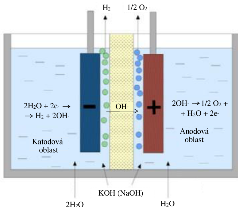
Obrázek 2.2 Schéma Alkalického elektrolyzéro [2]
