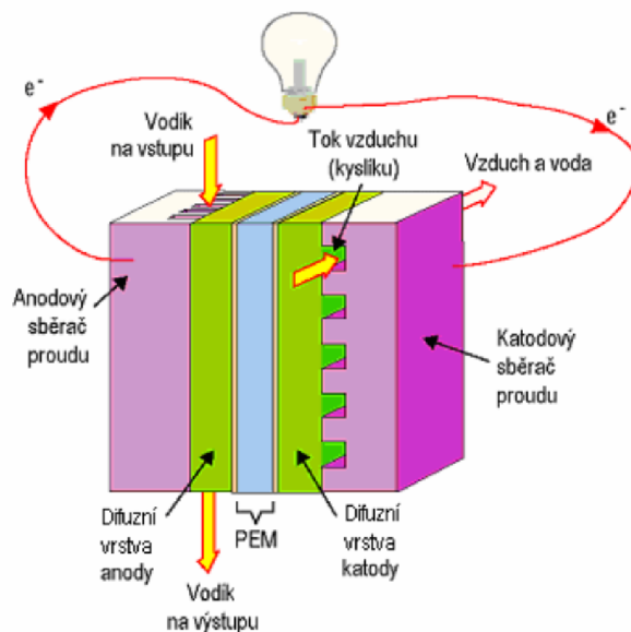
Obrázek 2.17 Elementární palivový článek s polymerní membránou [21]
