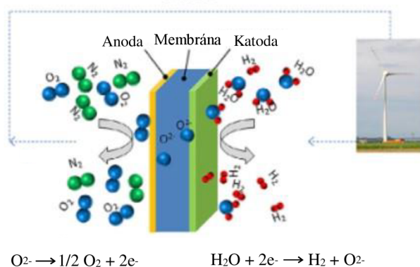
Obrázek 2.6 Schéma vysokoteplotního palivového článku a elektrolyzérů [7]
