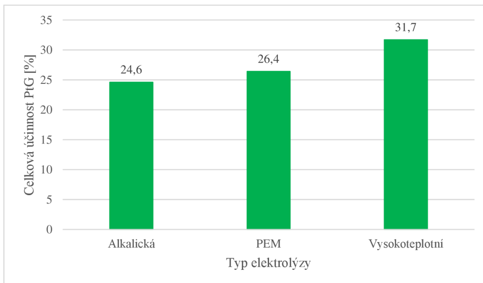
Obrázek 3.2 Vliv účinností jednotlivých typů elektrolyzérů na celkovou účinnost PtG
