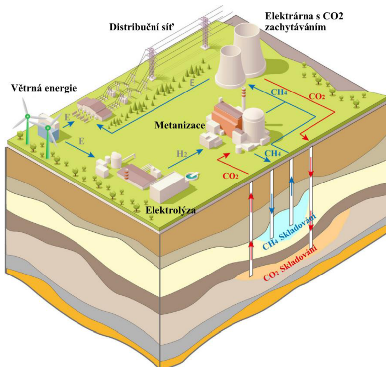
Obrázek 2.13 Skladování \text{CH}_4 a \text{CO}_2 v různých úložištích [17]
