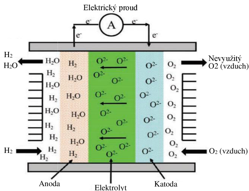
Obrázek 2.19 Schéma vysokoteplotního palivového článku [23]
