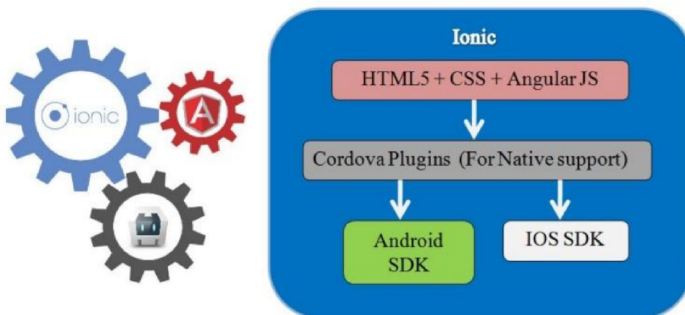
Obrázek 4: Architektura frameworku Ionic. Zdroj [4]
