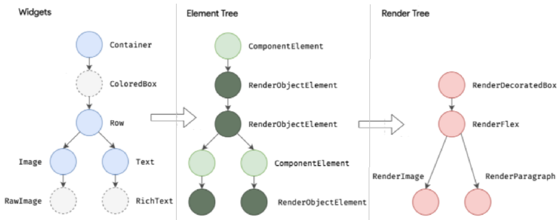
Obrázek 9: Postup při převádění widgetů do stromu prvků. Zdroj [6]
