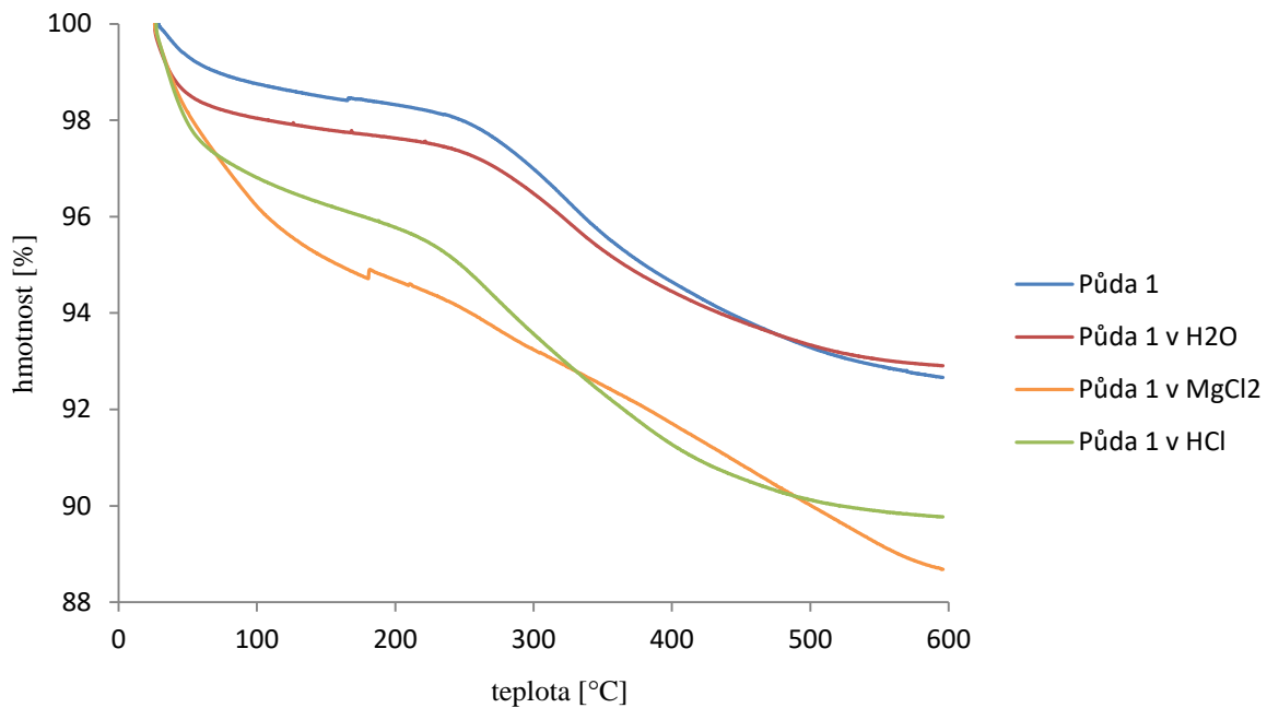
Obrázek 31: TGA křivky původní a extrahované půdy 1
