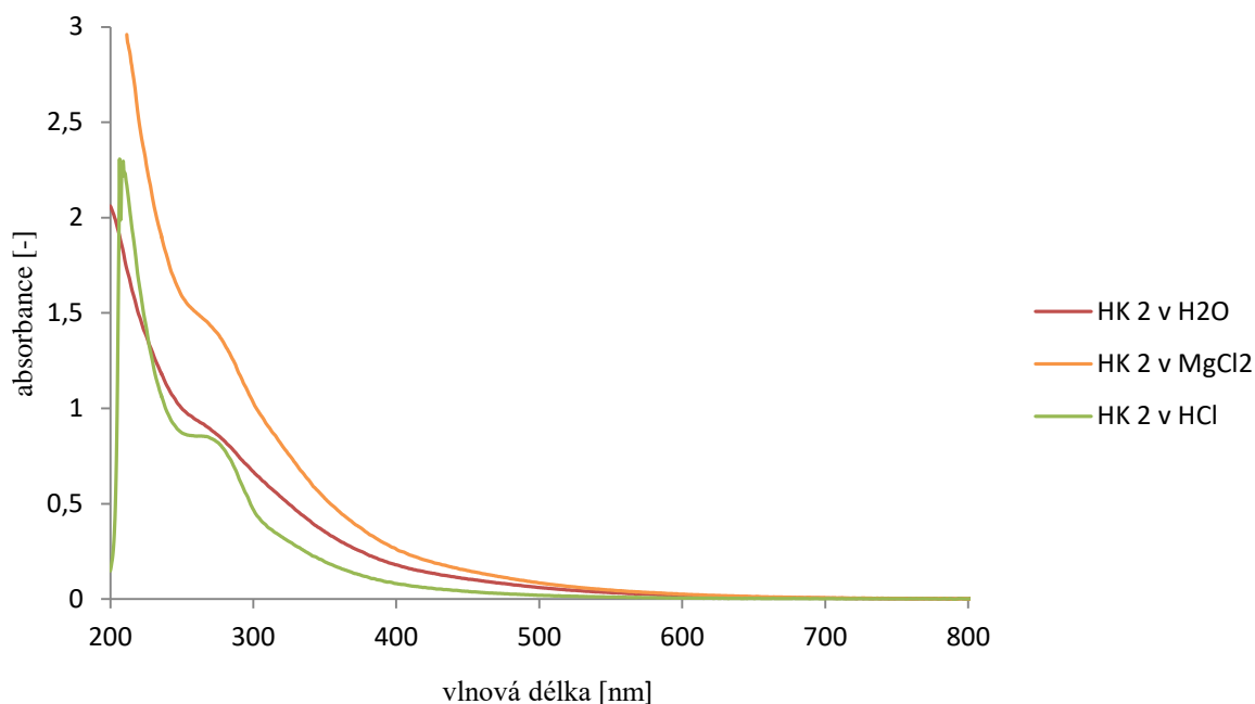
Obrázek 14: UV-VIS spektra výluhů huminové kyseliny 2
