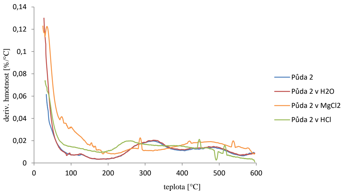
Obrázek 36: DTG křivky původní a extrahované půdy 2
