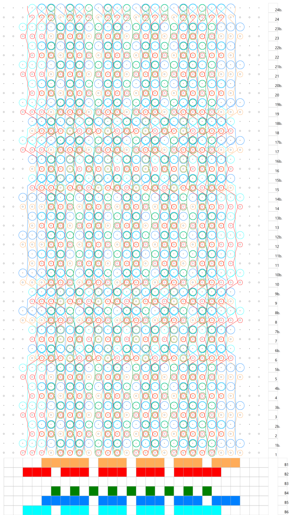
Obr. 19: Vazba 3 – 1x střída vzorové části pro jeden nosič
