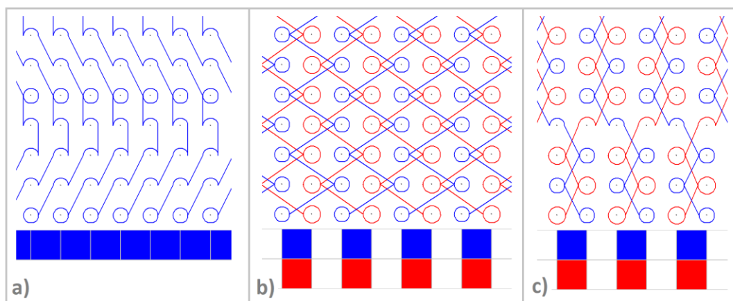
Obr. 4: Příklady filetových vazeb podle [26] - a) jedнопřístrojový filet, b) dvoupřístrojový filet v sukrové vazbě s malými otvory, c) dvoupřístrojový filet s velkými otvory
