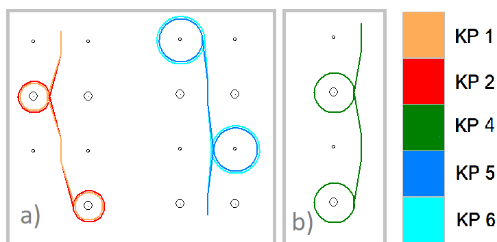
Obr. 13: Přechodová část – a) trikotové kladení pro KP 1, 2, 5, 6 (návlek 3:1); b) řetízkové kladení pro KP 4 (návlek 1:1)
