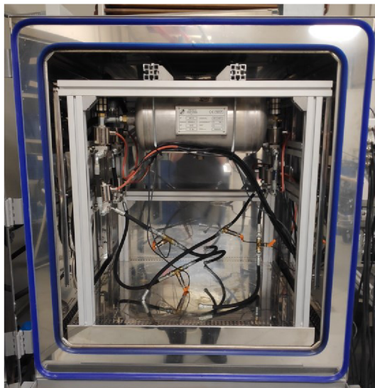
Obr. 2.20: Vnitřní prostor klimatické komory využívané ve zkušební společnosti Knorr-Bremse
