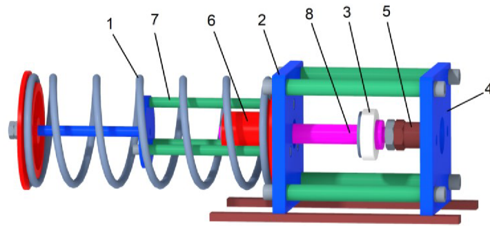
Obr. 2.21: Model stávajícího přípravku
