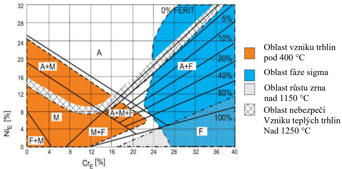
Obr. 20 Schaefflerův diagram [53].
