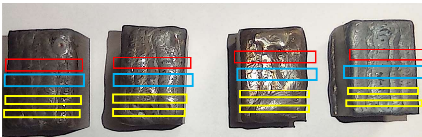
Obr. 26 Místa pro odběr vzorků makrostruktury, zleva vzorky A, B, C, D.
