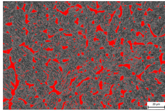
Obr. 56 Vyhodnocení podílu zbytkového austenitu pomocí ImageJ.
