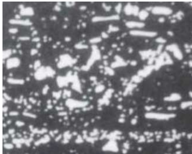
Obr. 19 Hrubá struktura s karbidickou řádkovitostí u PM-oceli [41].
