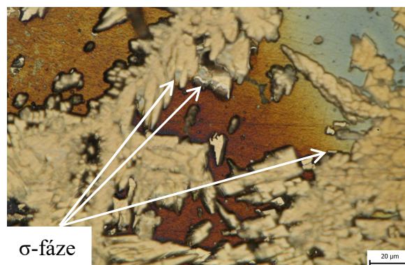
Obr. 46 Mikrostruktura MZV, vzorek A, zvětšení 200x, leptadlo Beraha.
