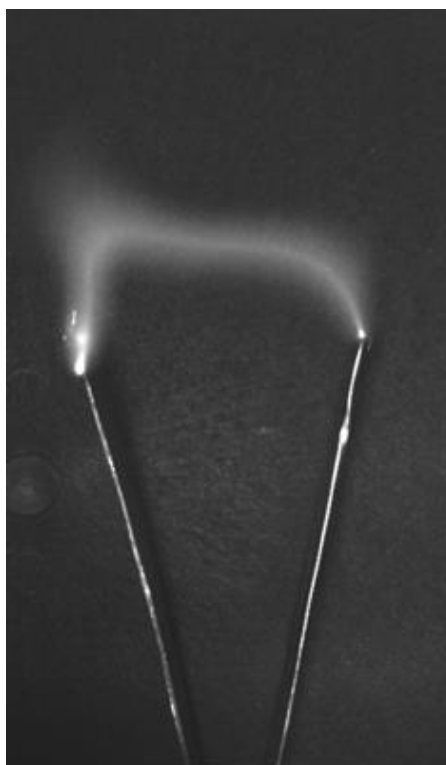
Obr. 22 Oblúk pri najväčšej vzdialenosti medzi elektródami
