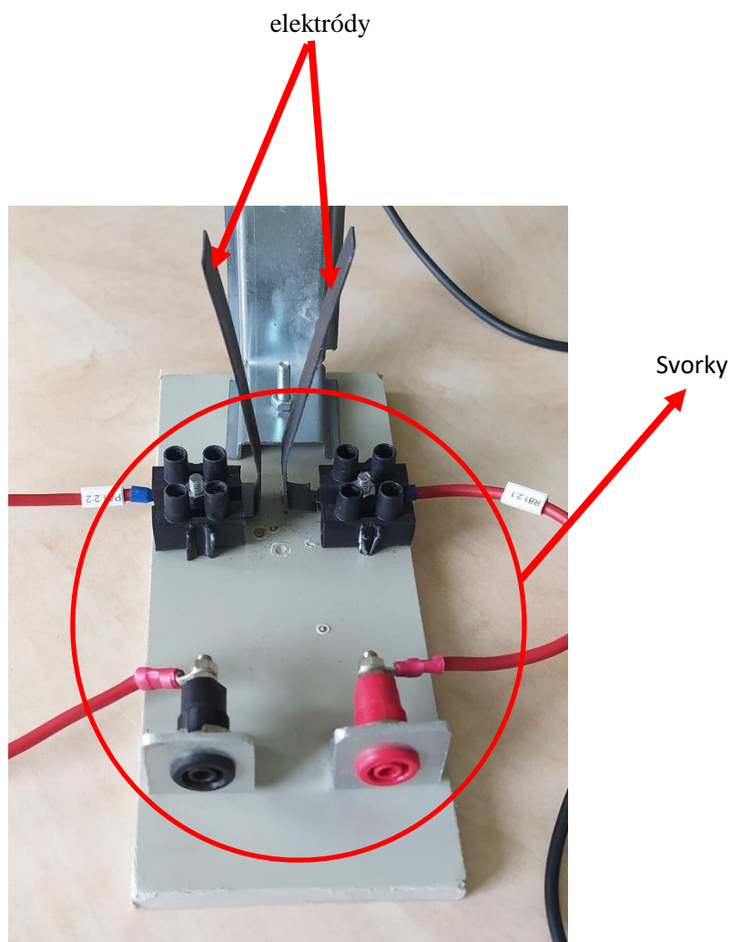
Obr. 5 Navrhnuté zariadenie
