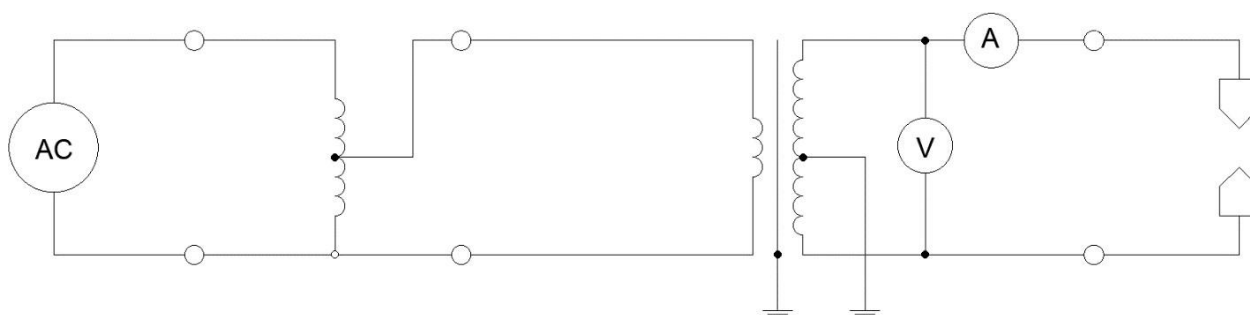
Obr. 18 Schéma merania
