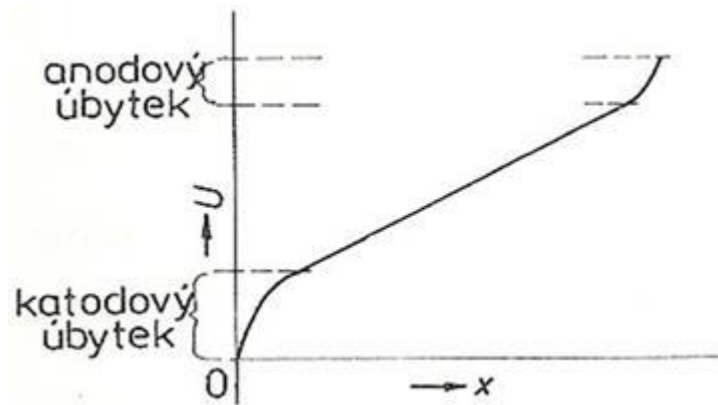
Obr. 2 Úbytky napätia na anóde a katóde pri horení oblúka [2]
