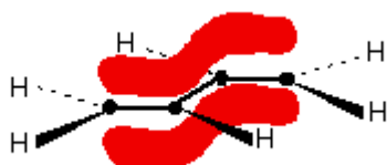
Obrázek 8: Delokalizace elektronu v buta-1,3-dienu.[18]
