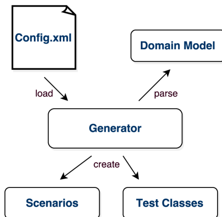
Obrázek 4.5: Koncept generátoru automatických testů.
