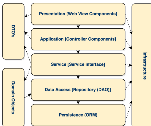
Obrázek 2.2: Architektura aplikace diagram [13].
