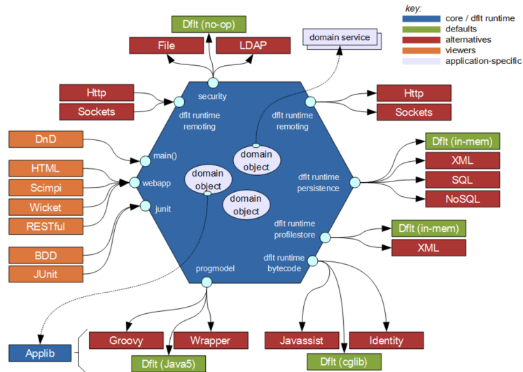
Obrázek 4.1: Hexagonální architektonický vzor [3].
