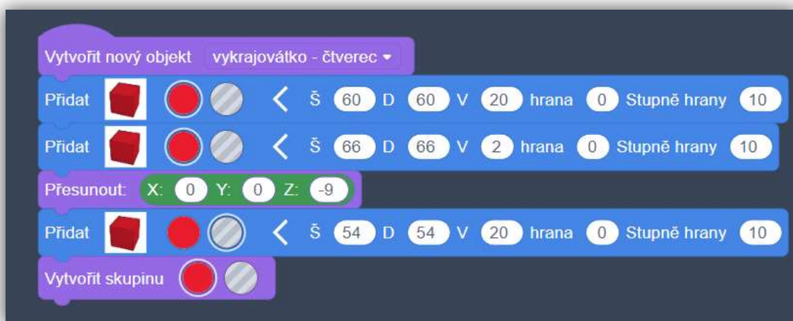
Obrázek 42: blokový kód pro výrobu vykrajovátko (Zdroj: vlastní zpracování)
