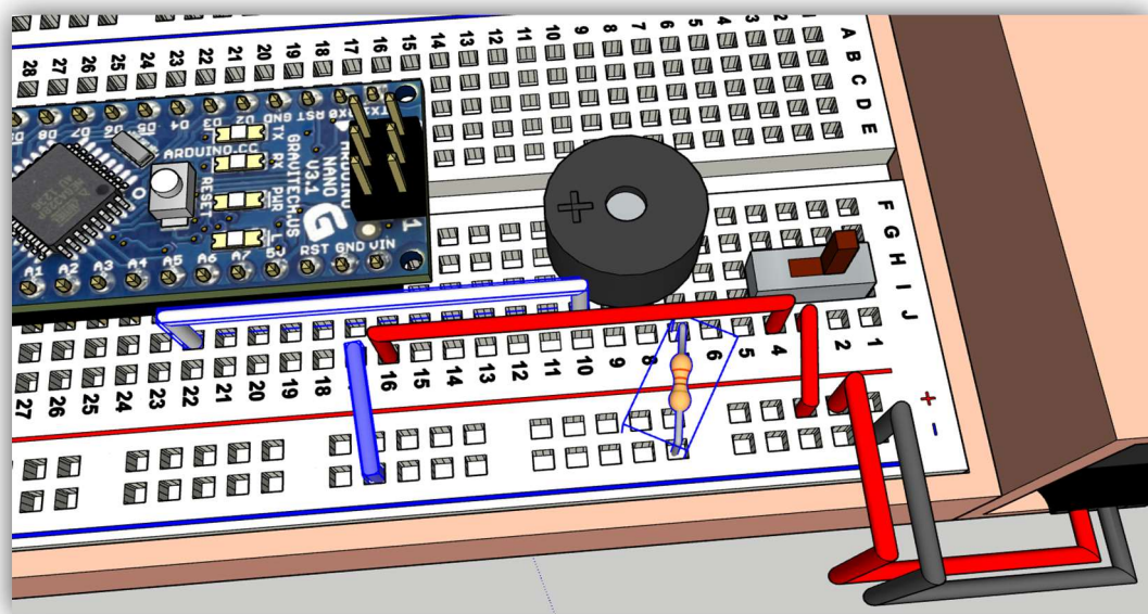
Obrázek 65: Reálné zapojení ultrazvuku
