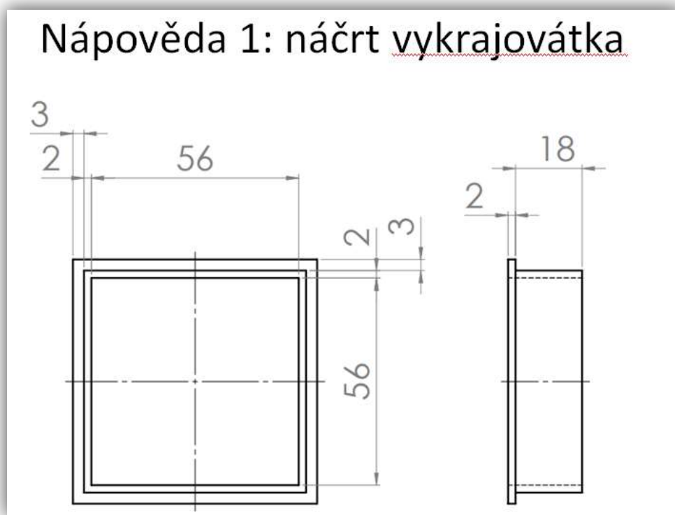
Obrázek 40: Náčrt vykrajovátko
