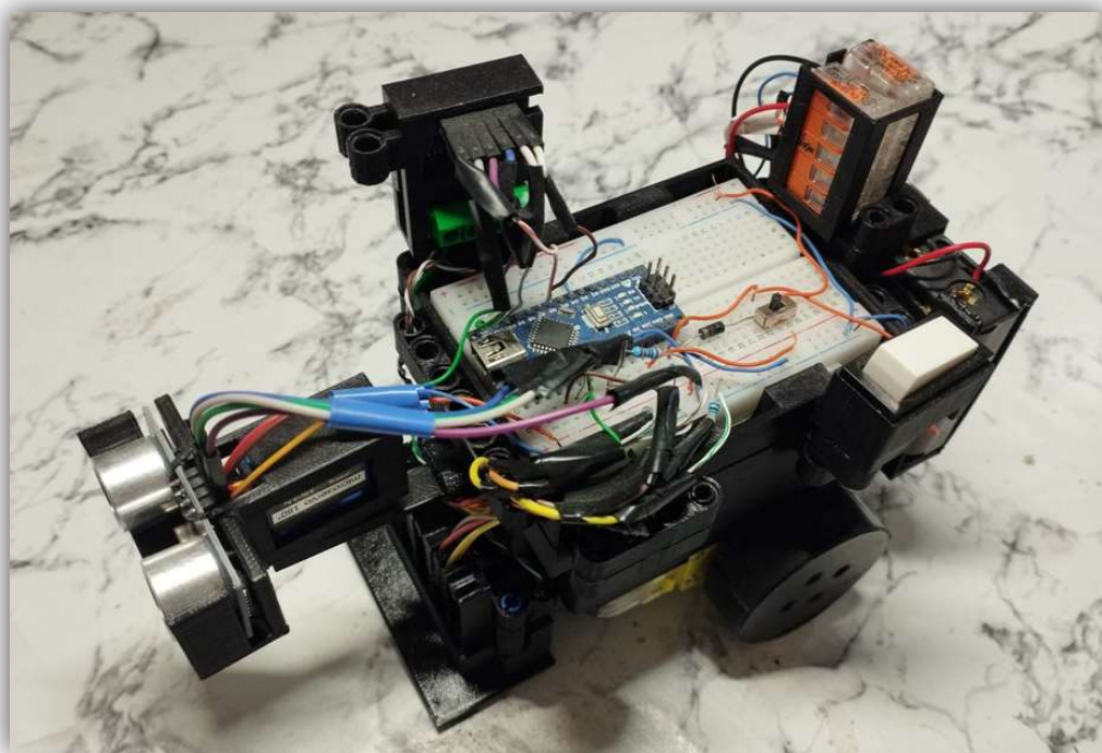
Obrázek 8: Robot řízený Arduinem
