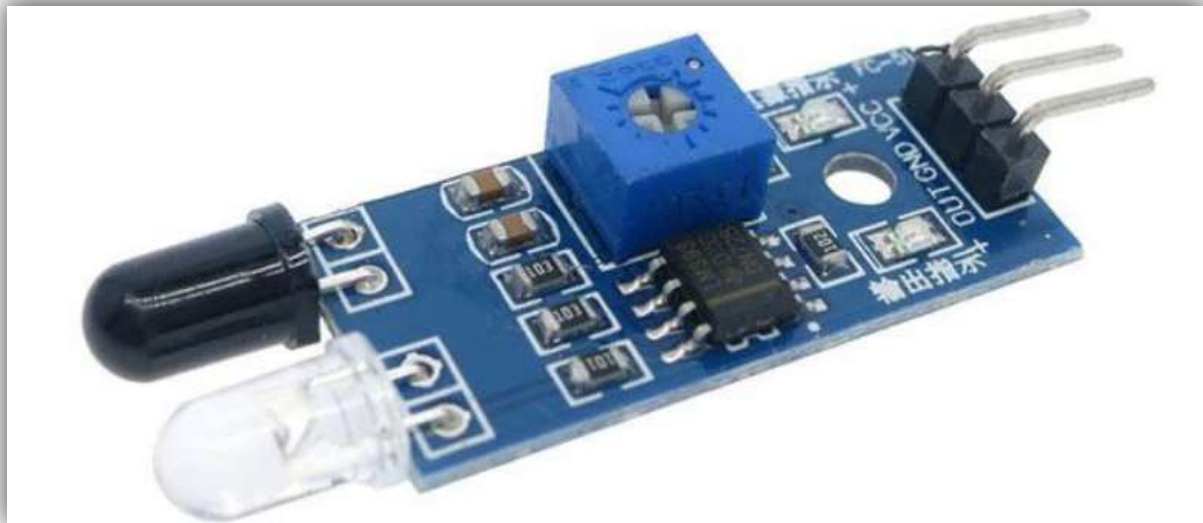
Obrázek 12: Reflexní světelná závora ( https://1url.cz/ergyJ )
