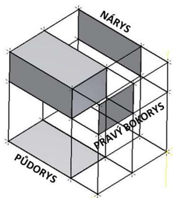
Obrázek 16: Technické kreslení
