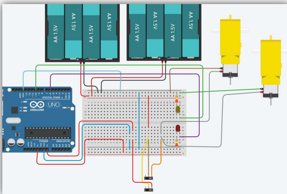
Obrázek 77: Postupné zapojování součástí v programu Sketchup (Zdroj: vlastní zpracování)
