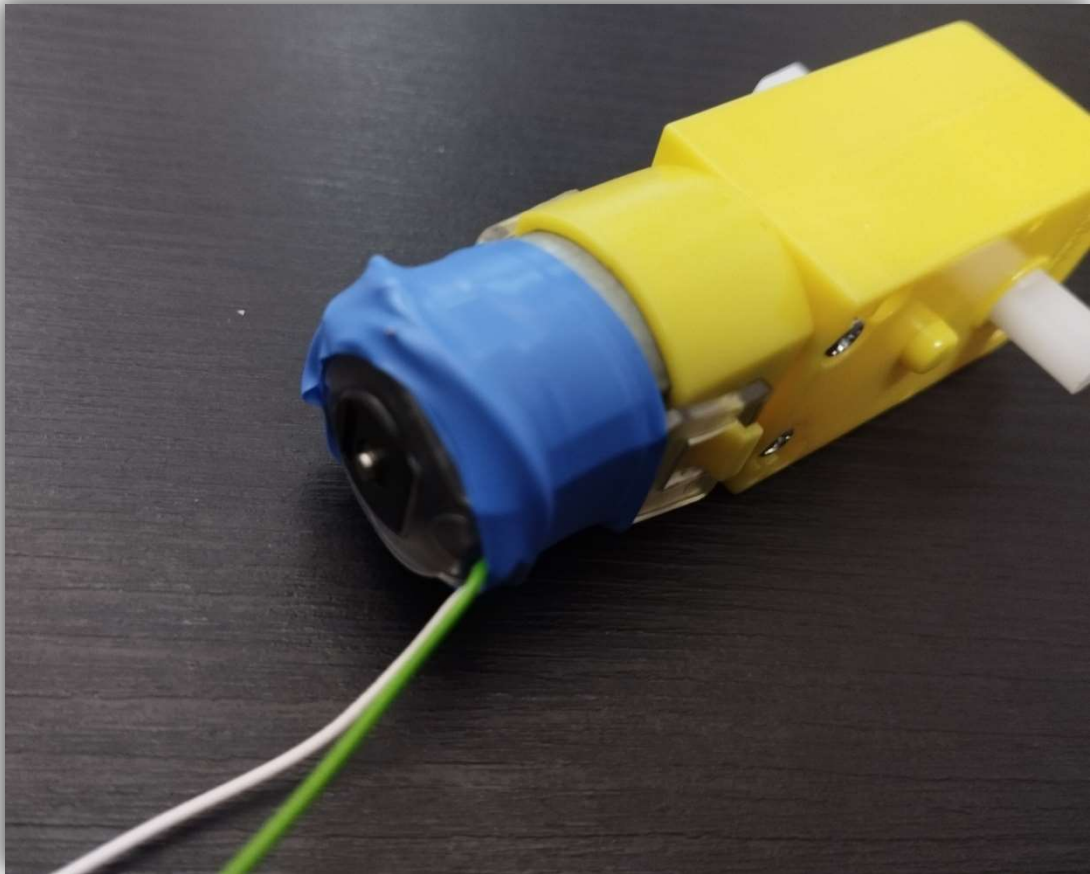
Obrázek 73: Předchystaný motor (Zdroj: vlastní fotoalbum)
