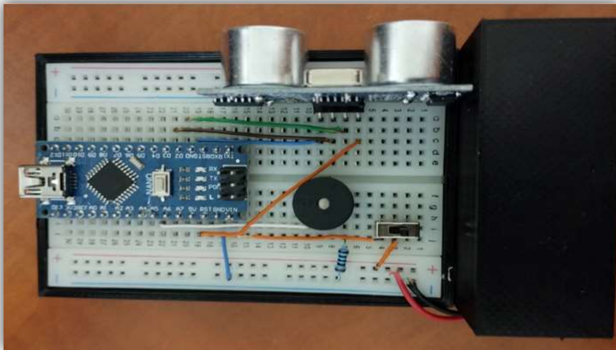
Obrázek 64: Zapojení elektrosoučástek
