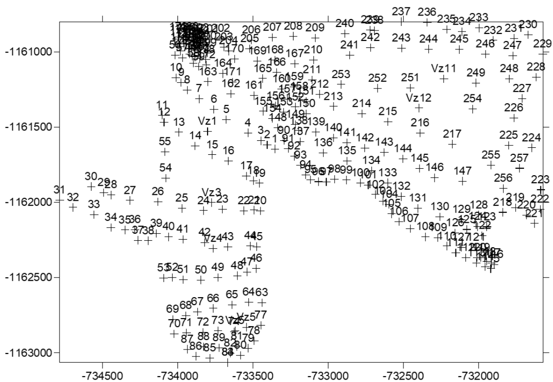
Obr. 4.2.3. Rybník Rožmberk – poloha bodů ve kterých byla měřena hloubka vody a mocnost sedimentu
