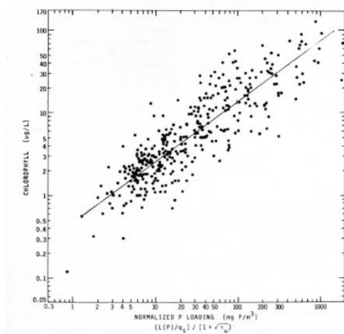
Obr. 2.1.1. Aktualizovaný Vollenweiderův OECD model vztahu mezi zatížením jezera fosforem a koncentrací chlorofylu v jezeře (Jones a Lee, 1986)
