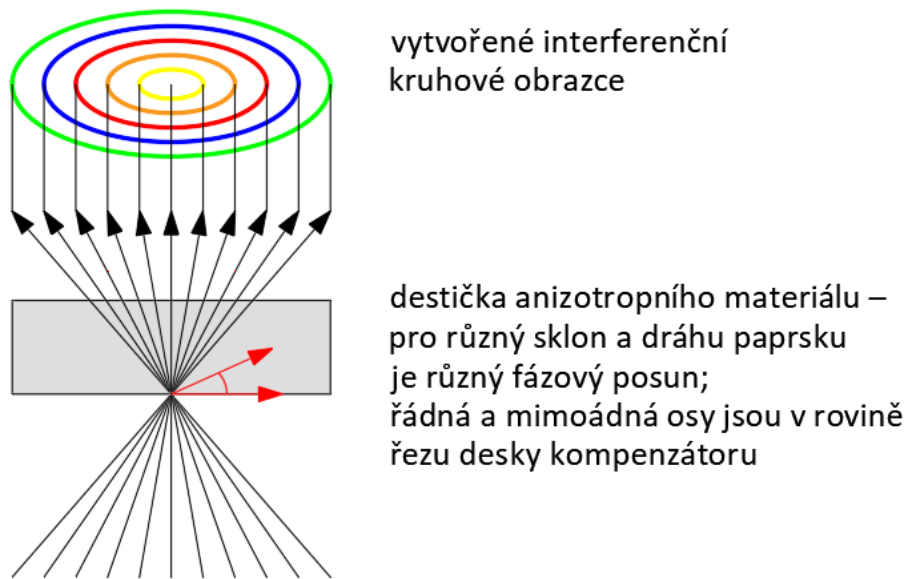
Obrázek 3: Vytváření intergefenčních kruhových obrazců
