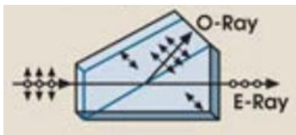
Obr. 41: Glan-Thompsonův polarizační hranol [25]
