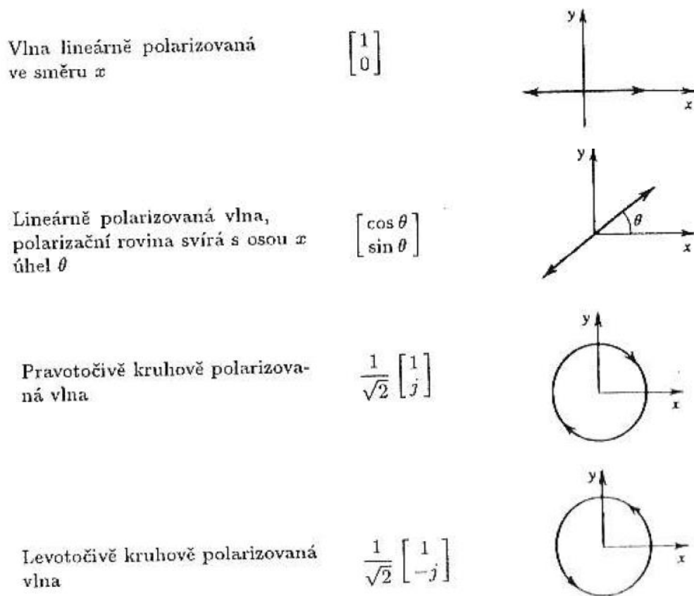
Obr. 18: Jonesovy vektory [2]
