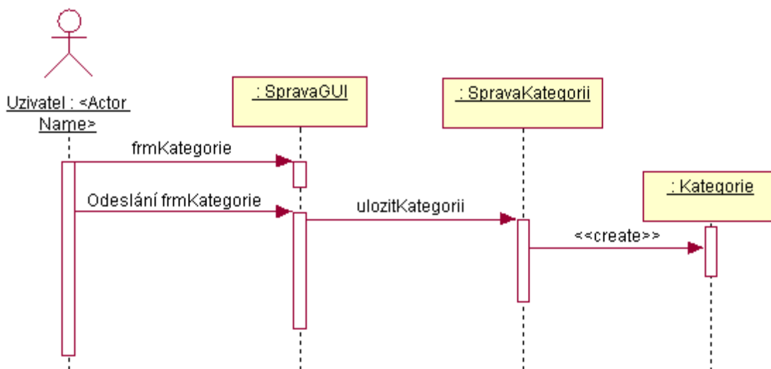
Obr. 6: Přidání nové kategorie
