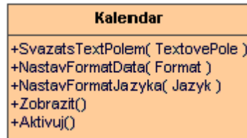
Obr. 20: Třída reprezentující ovládací prvek kalendář
