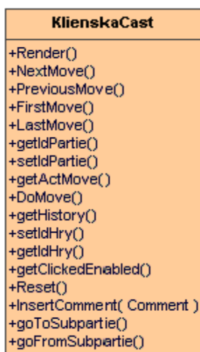
Obr. 17: Klientská část modulu
