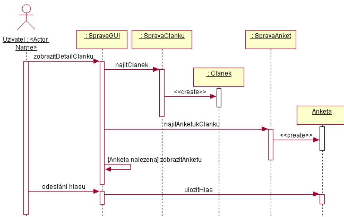
Obr. 9: Hlasování v anketách
