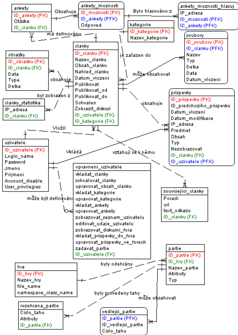
Obr. 22: Schéma databáze
