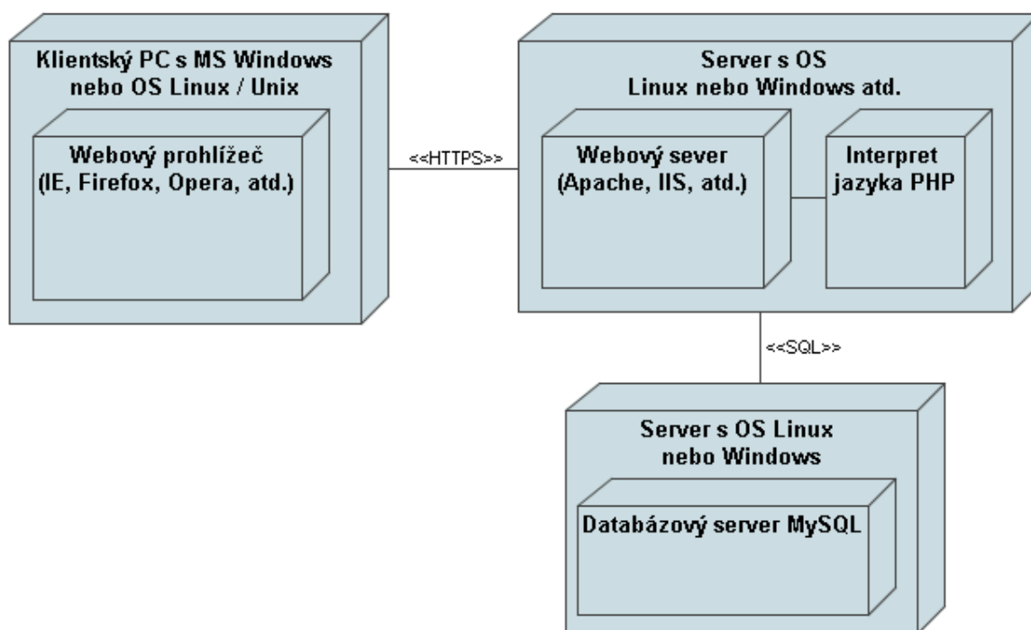
Obr. 18: Architektura systému
