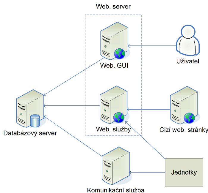
Obrázek 2.1: Architektura systému
