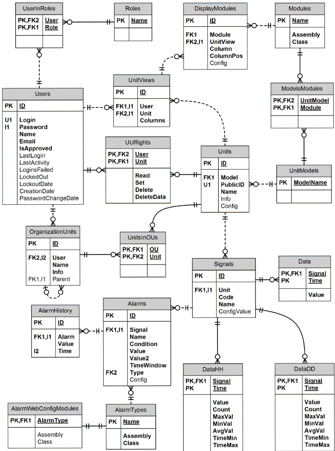
Obrázek 3.1: ER. diagram
