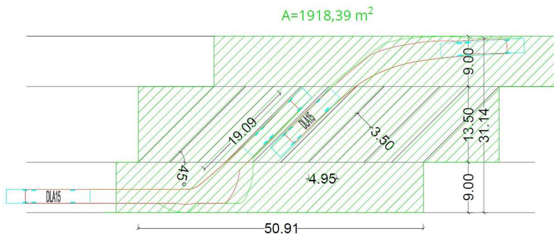
Obrázek 29: Plocha 10 stání s přilehlou komunikací, šikmé řazení 45°, rozměry stání ČSN 73 6056 (autobusy)
