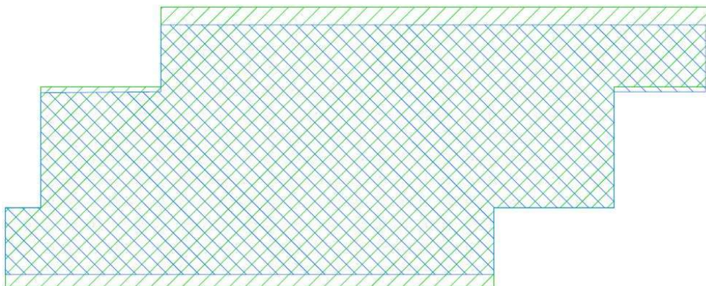
Obrázek 41: Grafické srovnání ploch parkovacích stání pro 10 vozidel, šikmé řazení 45^\circ (zelená ČSN 73 6056, modrá po optimalizaci, autobusy)
