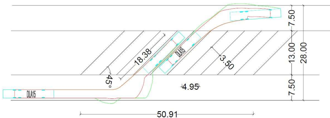
Obrázek 33: Vlečná křivka, šikmé řazení 45°, rozměry stání po optimalizaci (autobusy)
