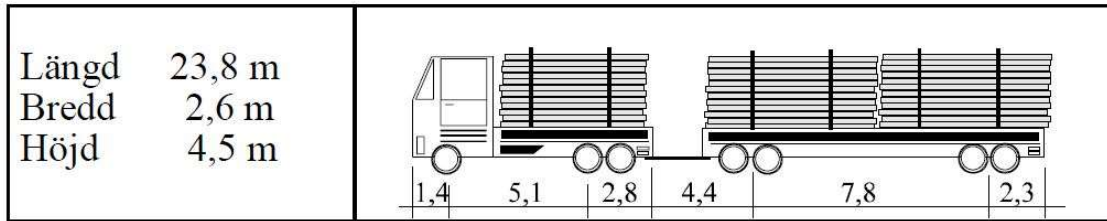
Obrázek 14: Skogsbil Ls [9]
