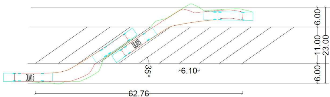
Obrázek 35: Vlečná křivka, šikmé řazení 35^\circ , nově navržená varianta stání (autobusy)
