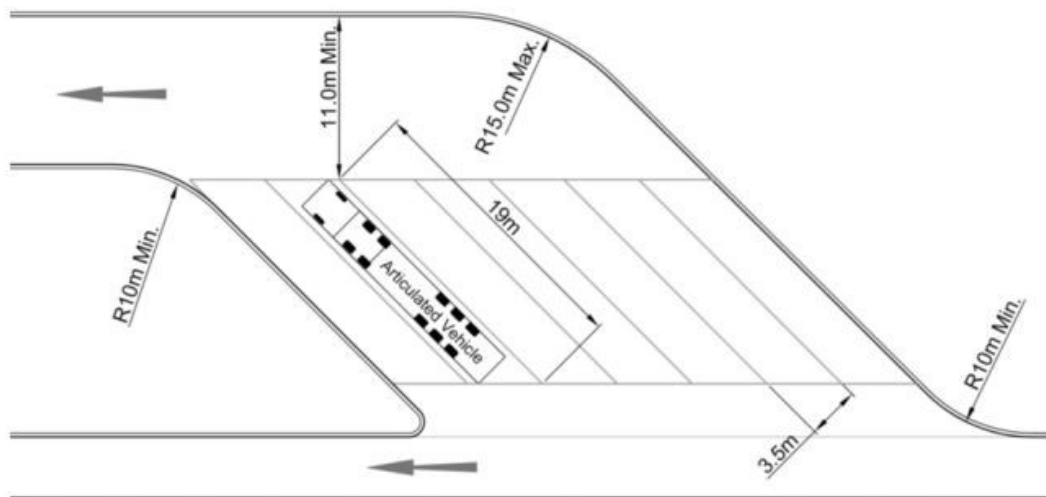
Obrázek 17: Jednosměrný parkovací systém se zálivy úhlu 45° pro nákladní automobily [12]
