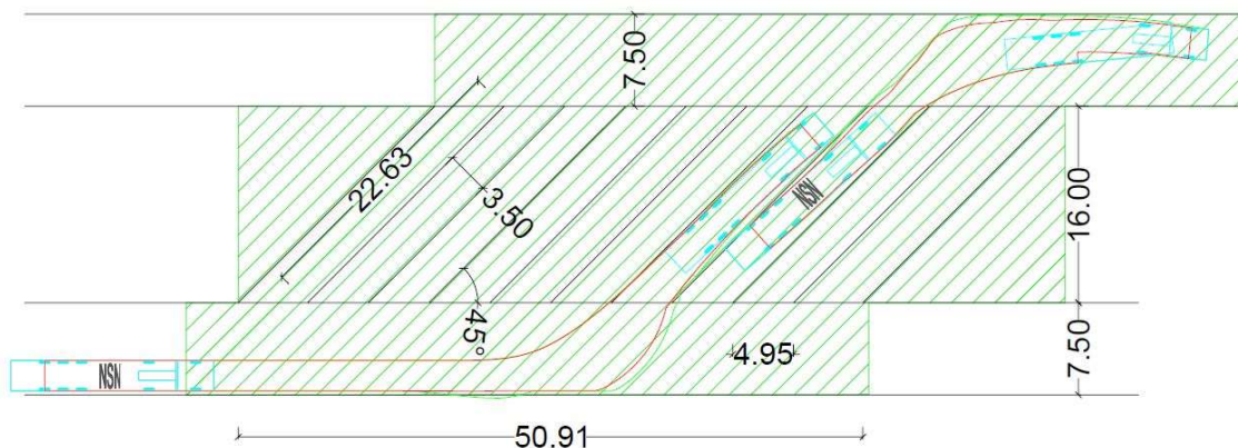
Obrázek 53: Plocha 10 stání s přilehlou komunikací, šikmé řazení 45°, rozměry stání ČSN 73 6056 (nákladní automobily)
