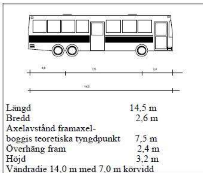
Obrázek 8: Boggibuss Bb [9]
