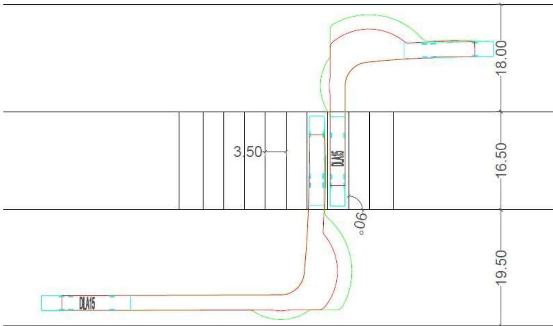
Obrázek 21: Vlečná křivka, kolmé parkování, rozměry stání ČSN 73 6056 (autobusy)
