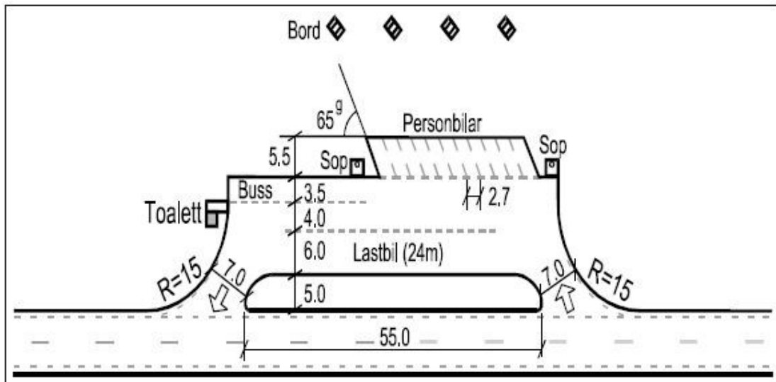
Obrázek 15: Příkladný návrh odpočívky s jedním jízdním pruhem [10]
