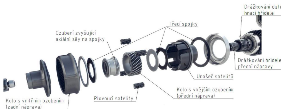
Obrázek 22 Audi Self-locking center differential: popis součástí [29]
