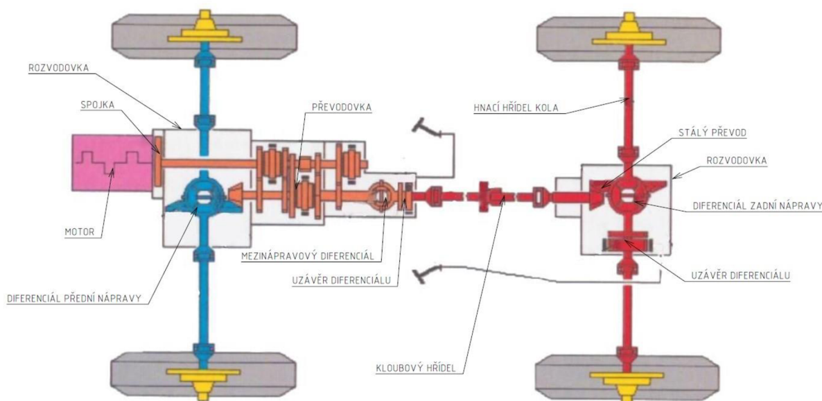
Obrázek 1 Převodové ústrojí automobilu [1]
