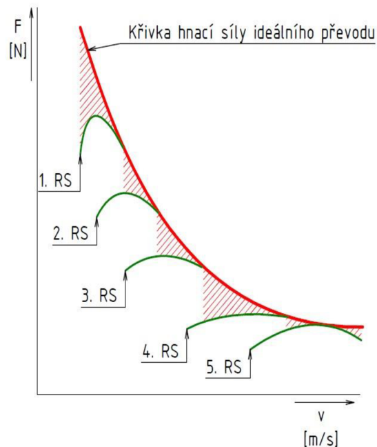
Obrázek 4 Graf hnacích sil rychlostních převodů a hnací síly ideálního převodu
