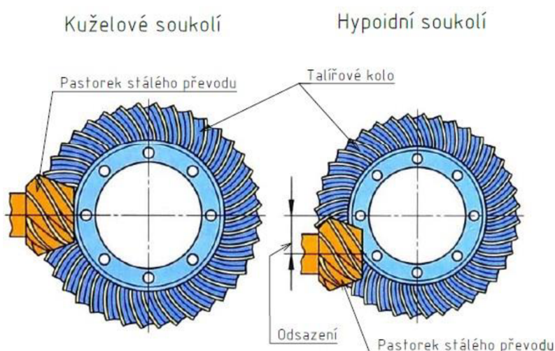
Obrázek 5 Porovnání Kuželového a Hypoidního soukolí [35]
