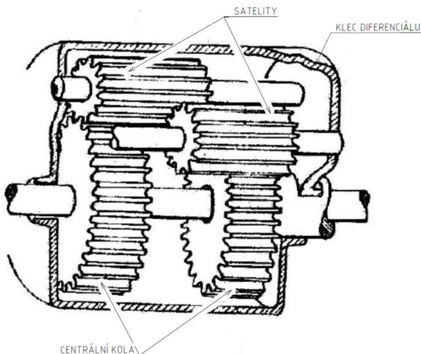
Obrázek 8 Popis částí otevřeného čelního diferenciálu [5]
