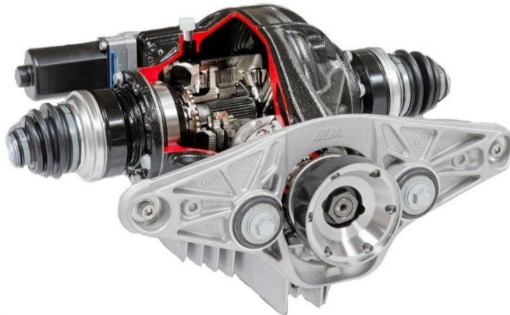
Obrázek 14 Aktivní M diferenciál [11]
