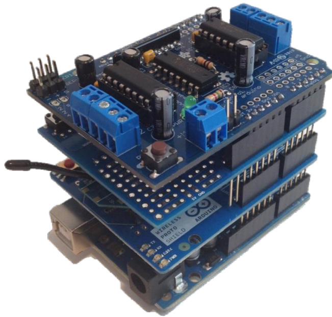
Obrázek 3- Arduino shieldy naskládáné na sebe
