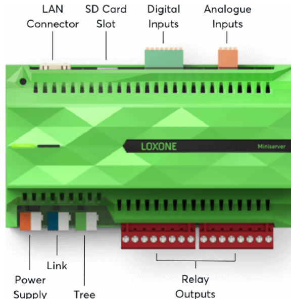
Obrázek 7- Miniserver Loxone s popisem
