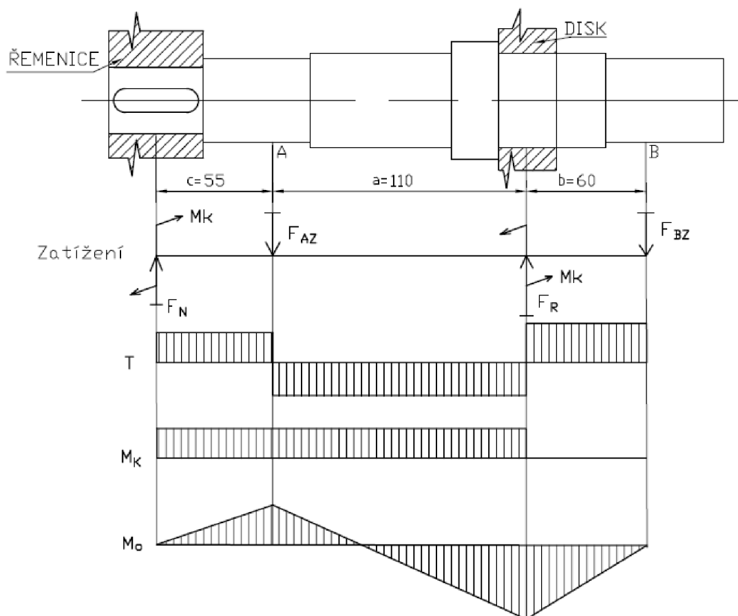
Obr. 28 Průběh VVÚ na hřídeli drtičeho mechanismu – rovina XZ
