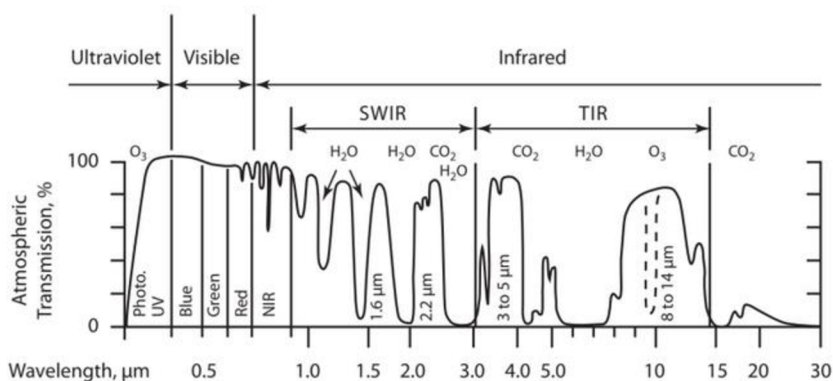
Obrázek 3 - Propustnost atmosféry [12]
