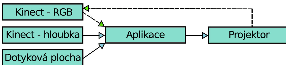
Obrázek 5.1: Schéma systému. Aplikace zpracovává data ze vstupů a výsledek promítá na stůl. Při kalibraci Kinectu aplikace zpracovává i barevný obraz tím vzniká zpětná vazba (přerušovaná zelená šipka).
