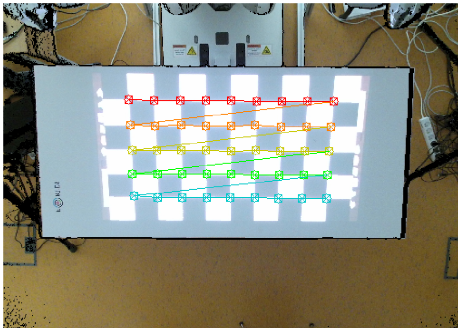
Obrázek 6.3: Ukázka barevného obrazu z Kinectu namapovaného na hloubková data pořizovaného během kalibrace Kinectu. Do obrazu jsou vykresleny nalezené vnitřní rohy šachovnice.
